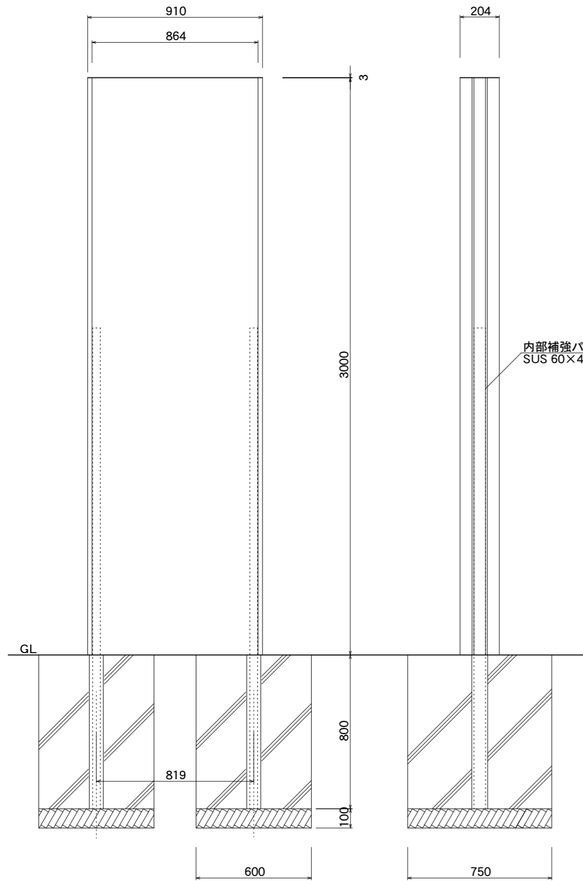
【正面図】
