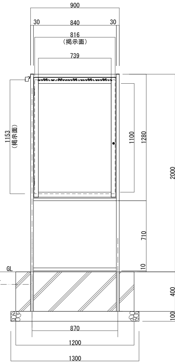
【正面図 S=1:20】
