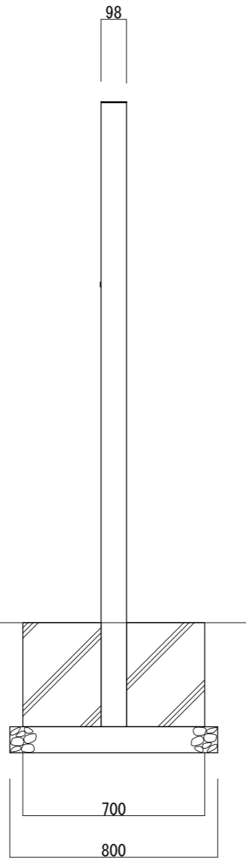
【側面図 S=1:20】
