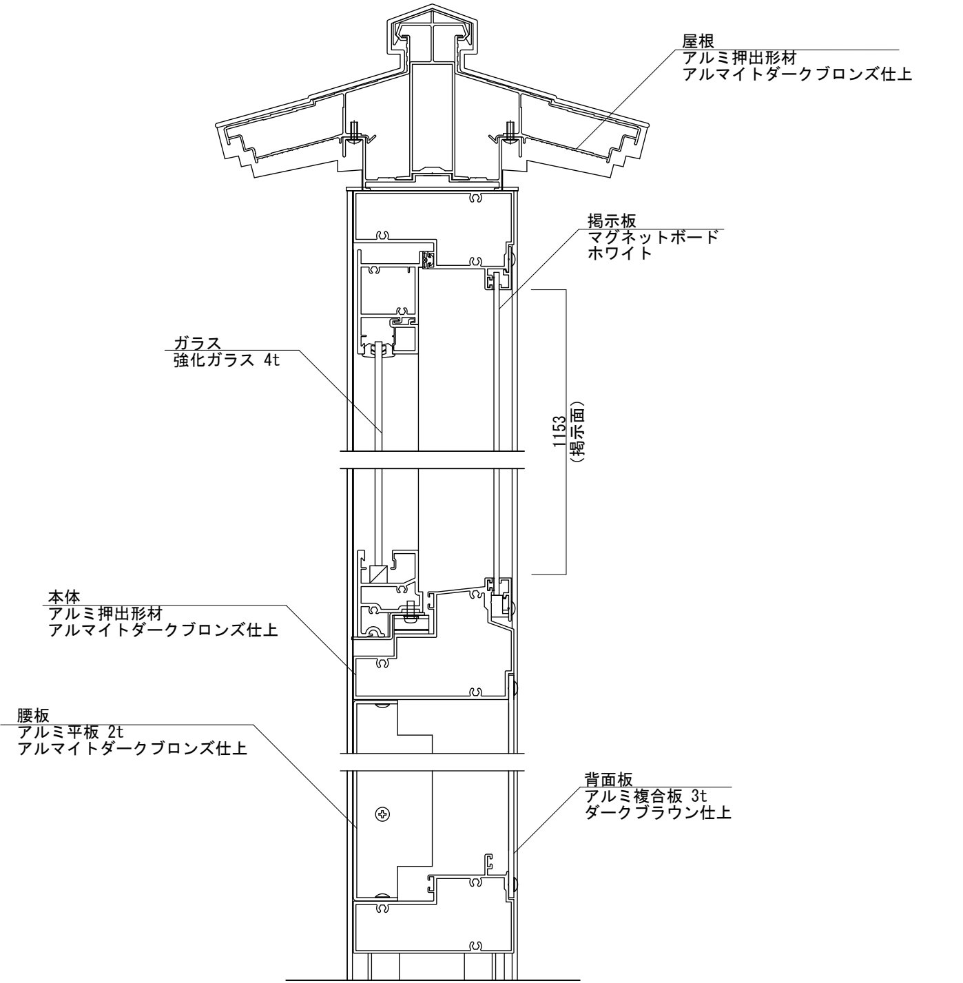
【側断面図 S=1:3】
