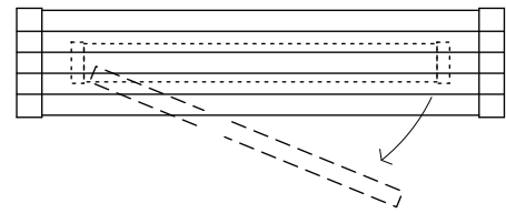
【平面図 S=1:20】
