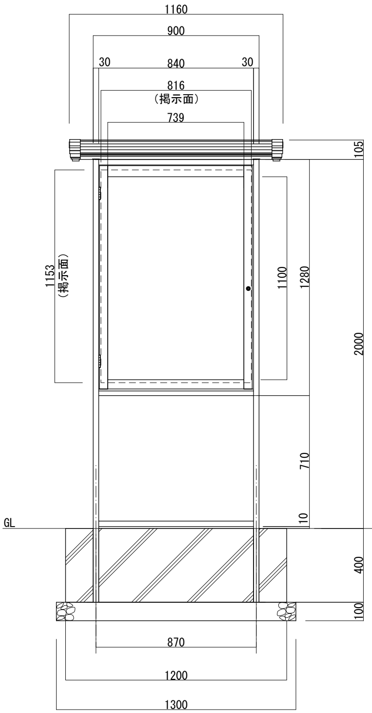
【正面図 S=1:20】
