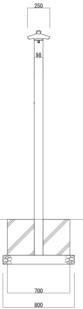
【側面図 S=1:20】
