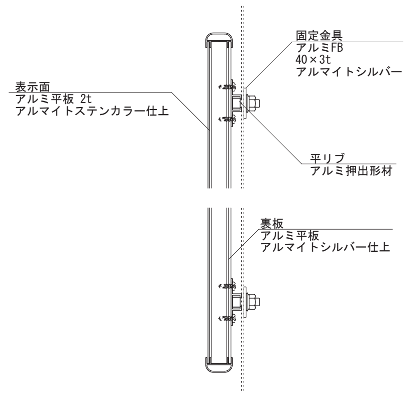
【側面図 S=1:5】
