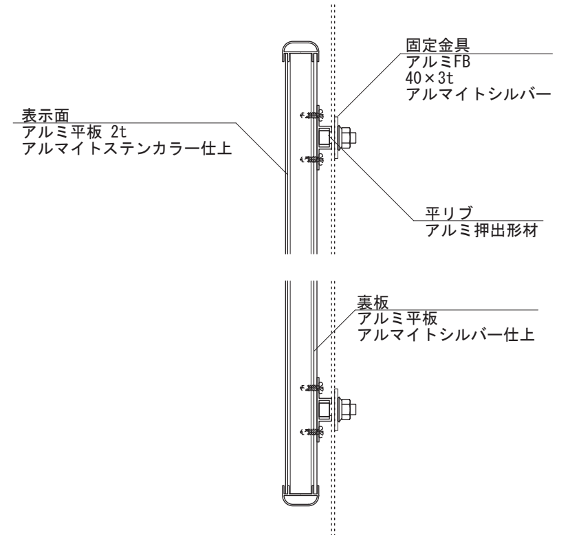
【側面図 S=1:5】
