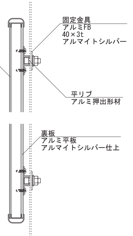
【側面図 S=1:5】
