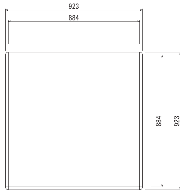
【正面図 S=1:15】
