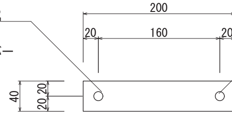
【固定金具加工図 S=1:5】
