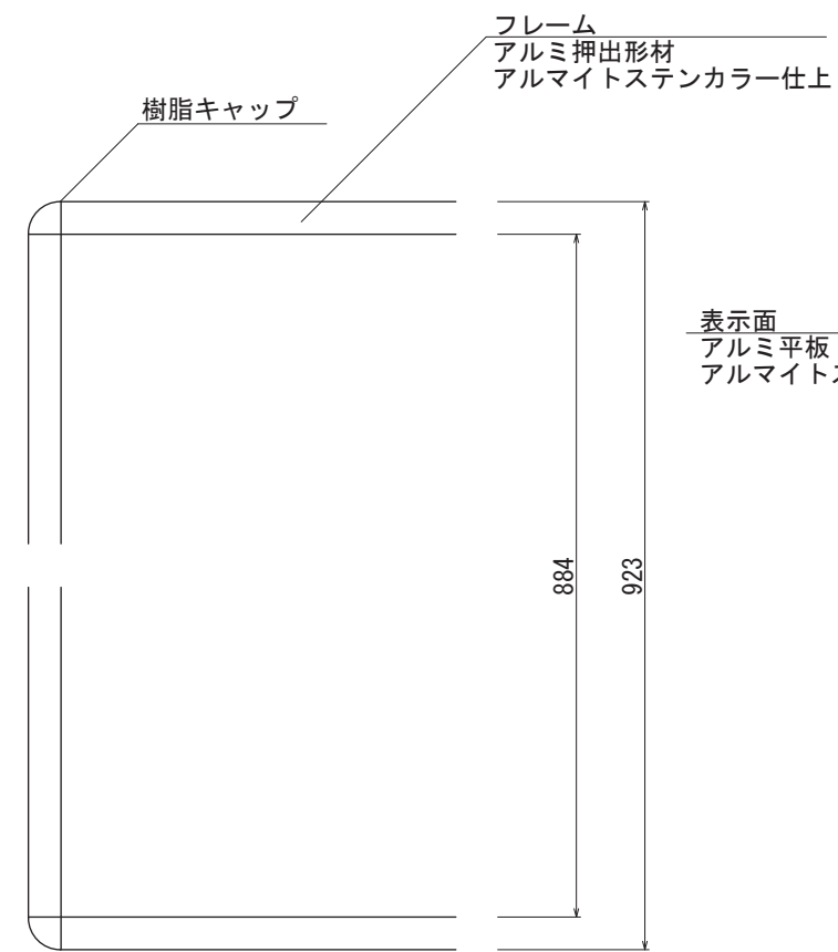
【平面図 S=1:5】
