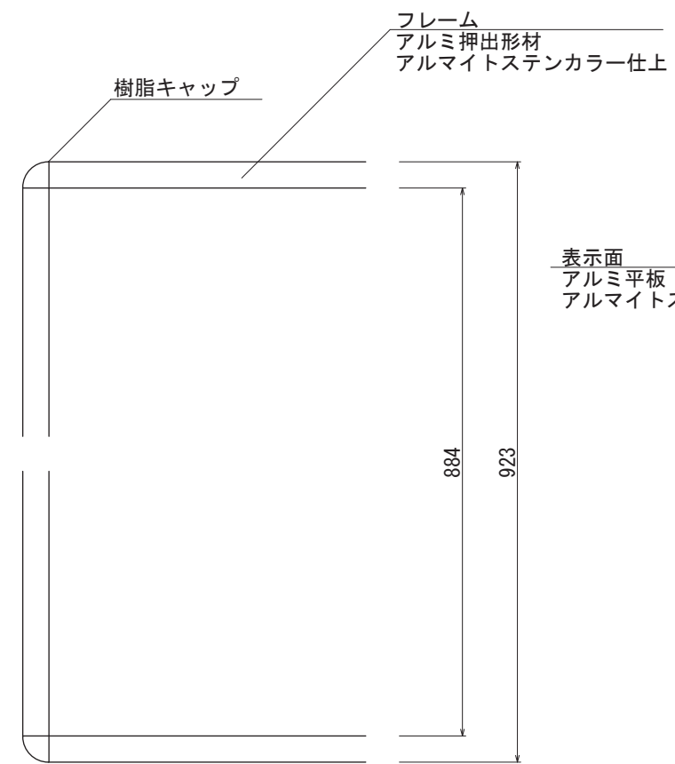
【平面図 S=1:5】
