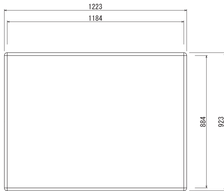
【正面図 S=1:15】
