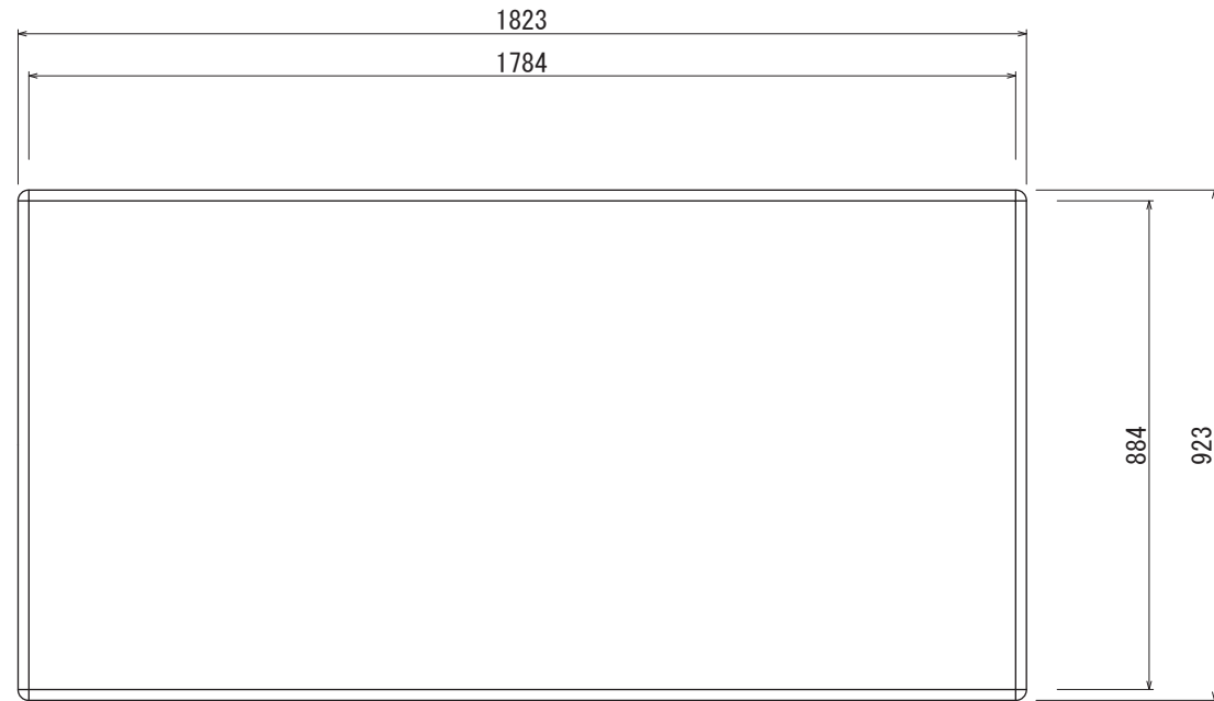
【正面図 S=1:15】
