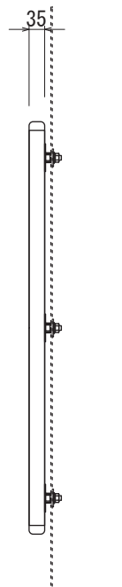
【側面図 S=1:15】
