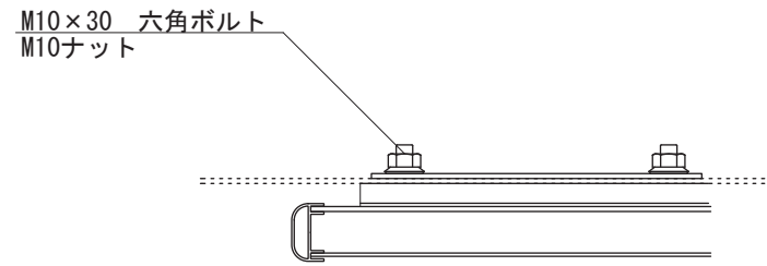
【平面図 S=1:5】
