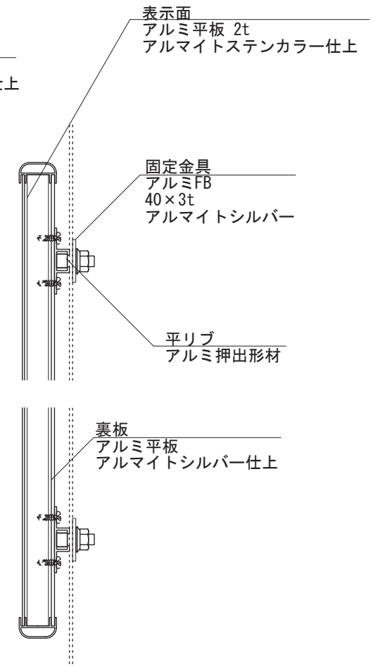
【側面図 S=1:5】
