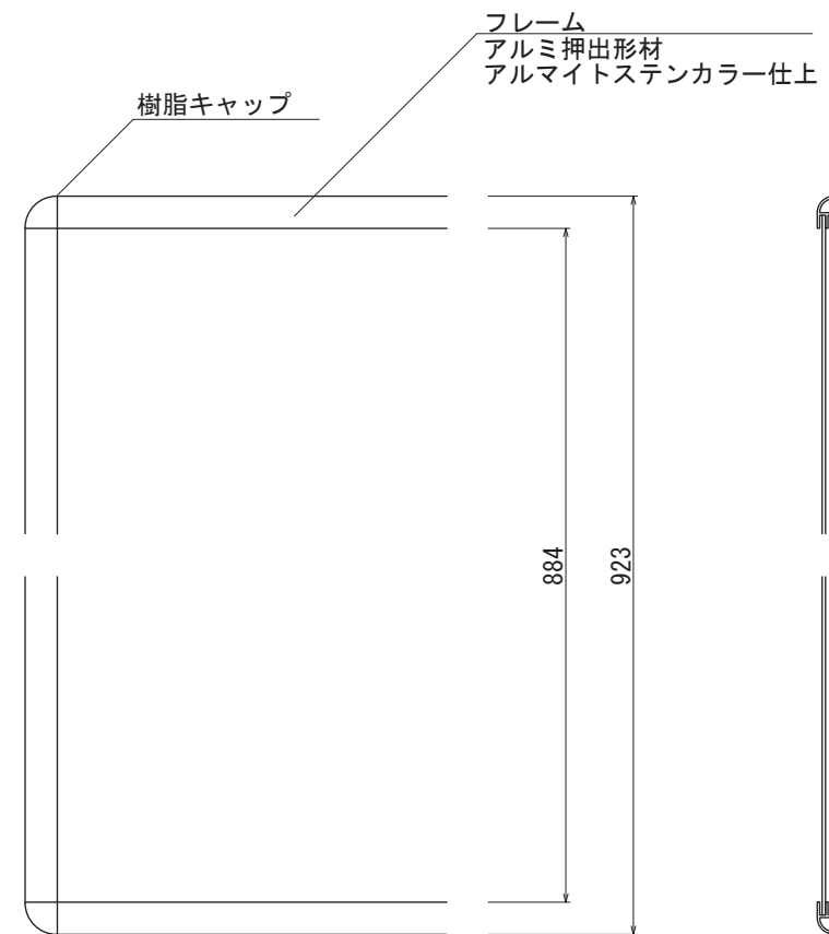
【平面図 S=1:5】
