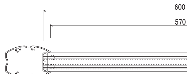
【平面図 S=1:5】
