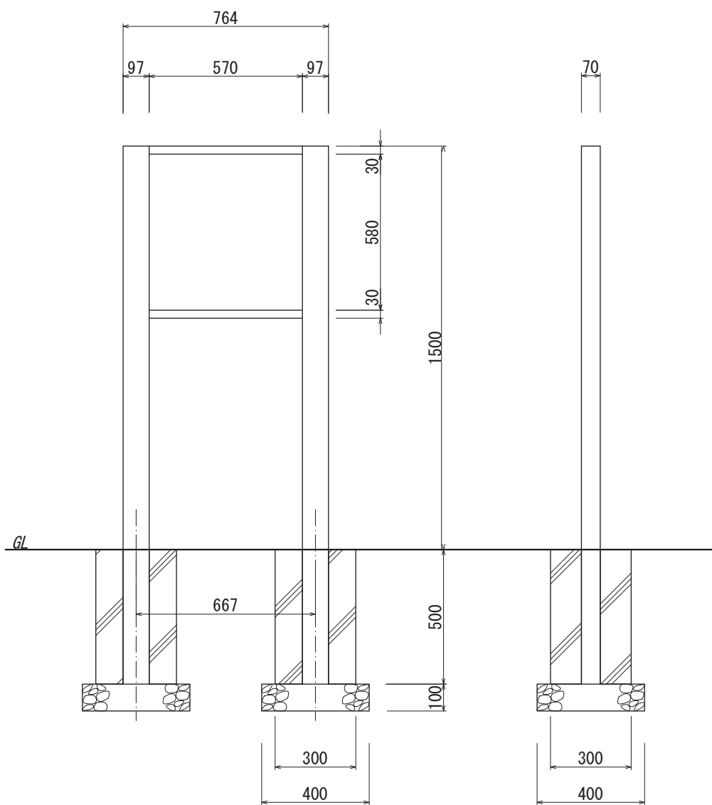
【正面図 S=1:20】
