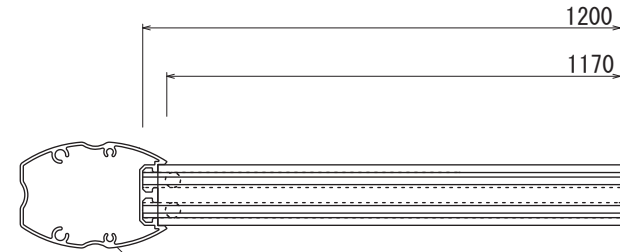
【平面図 S=1:5】
