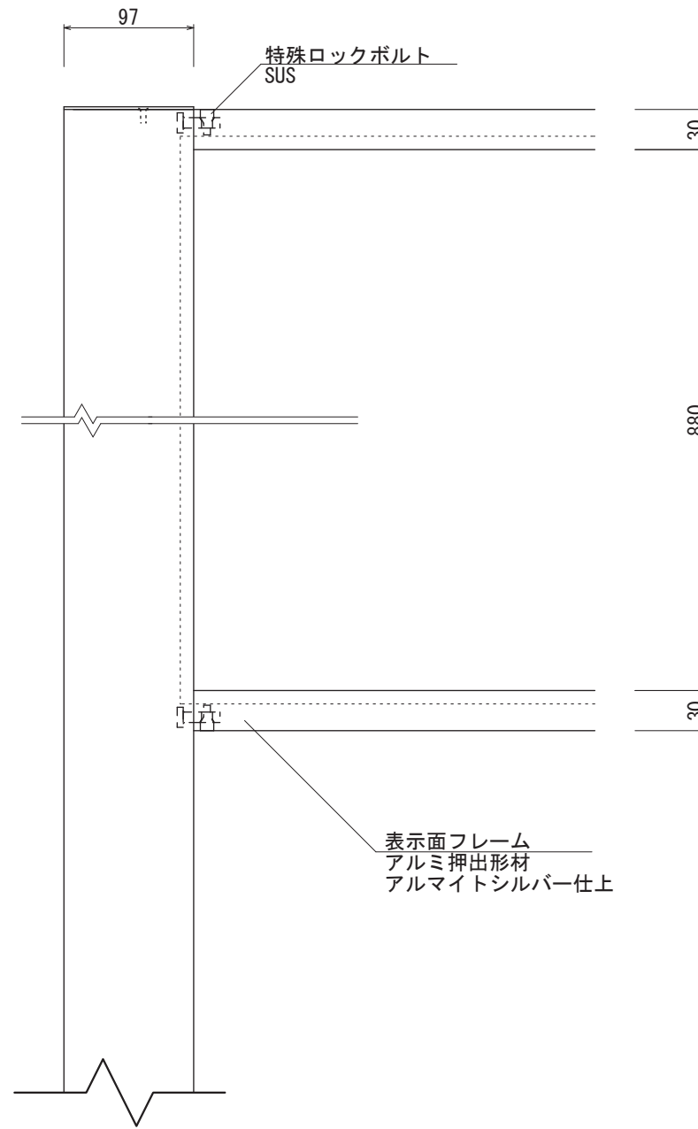
【正面図 S=1:5】
