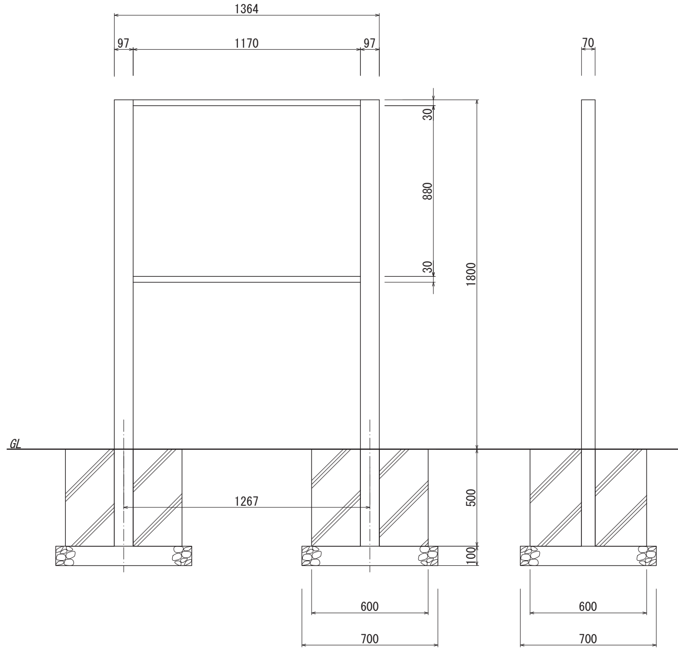
【正面図 S=1:20】
