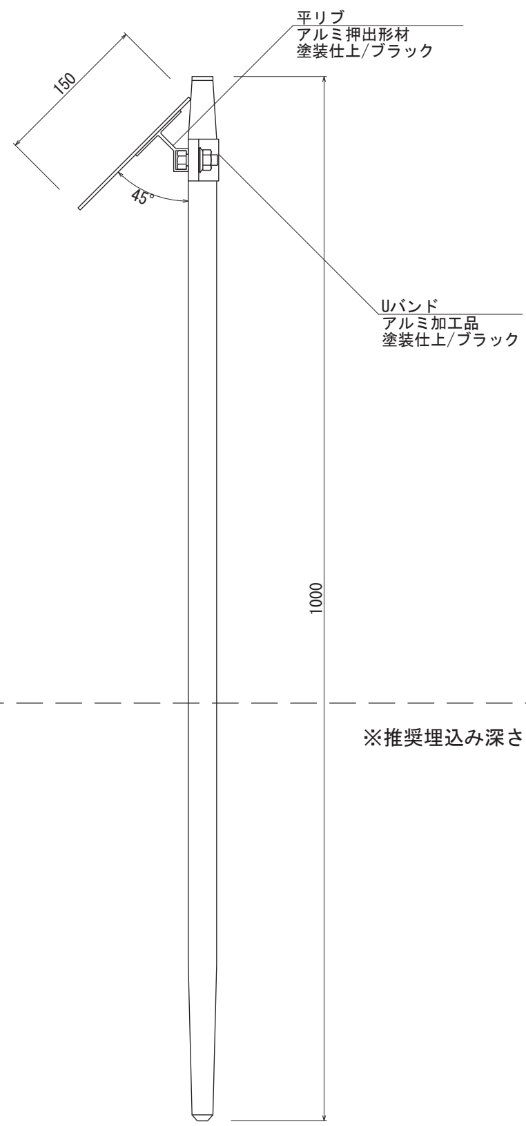
【側面図 S=1:5】
