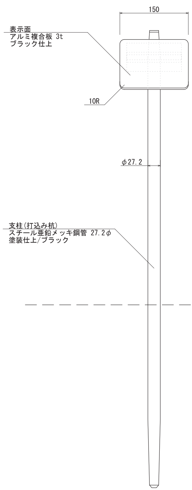
【正面図 S=1:5】
