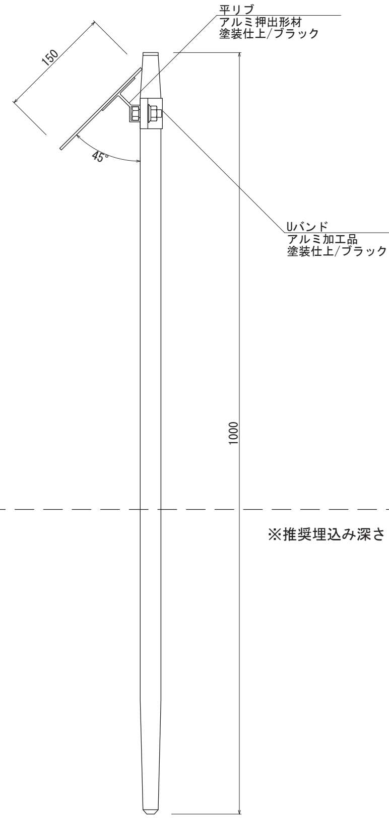
【側面図 S=1:5】
