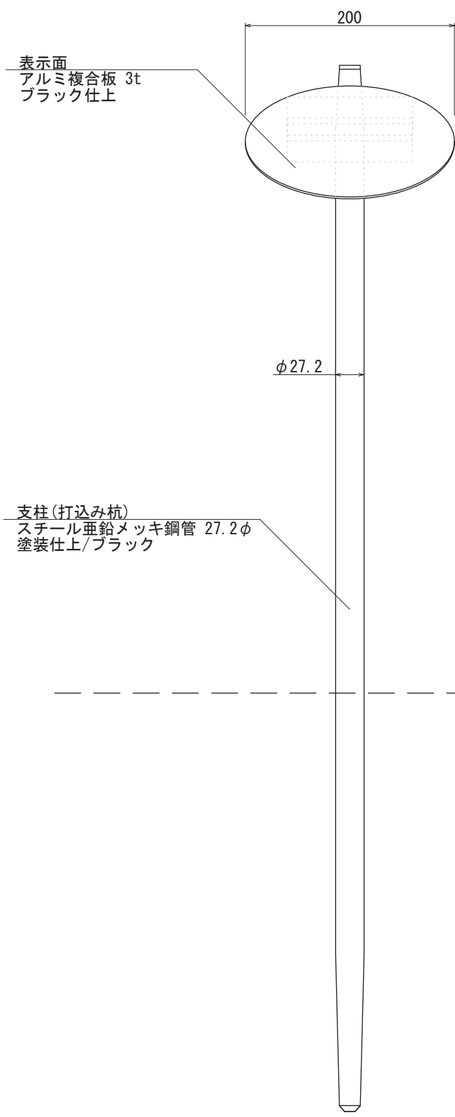
【正面図 S=1:5】
