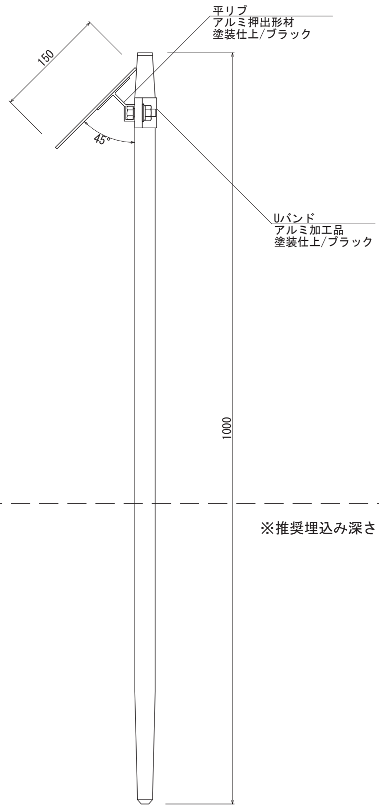
【側面図 S=1:5】
