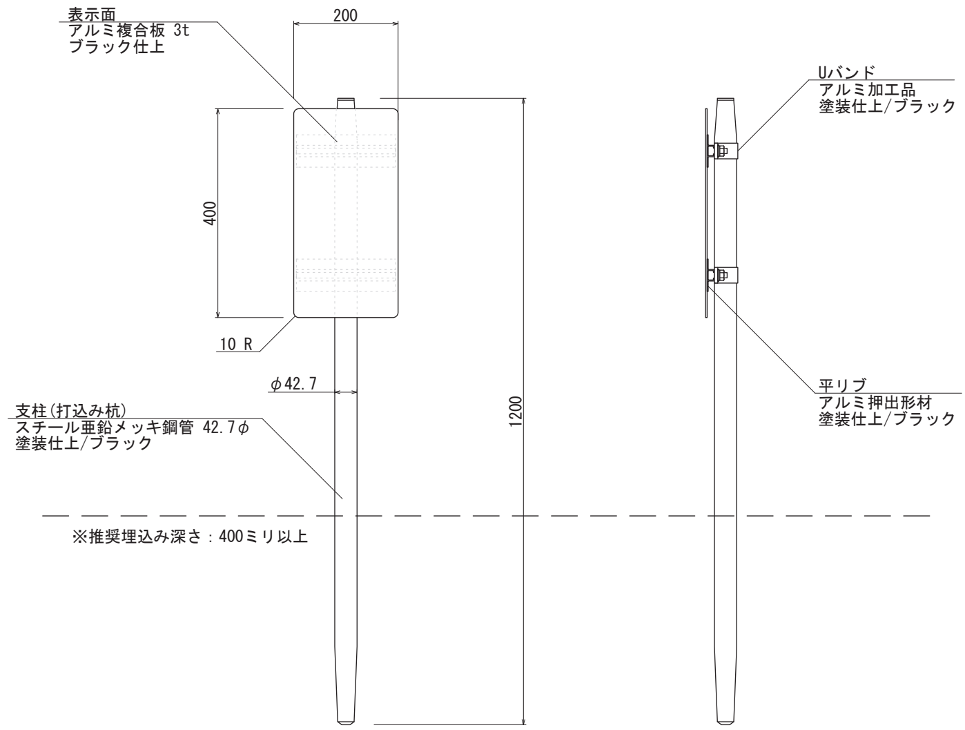
【正面図 S=1:10】
