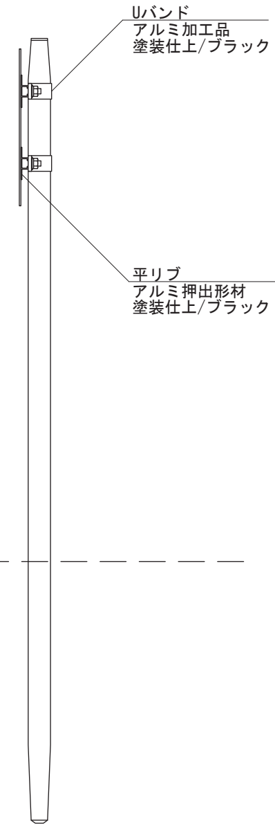
【側面図 S=1:10】
