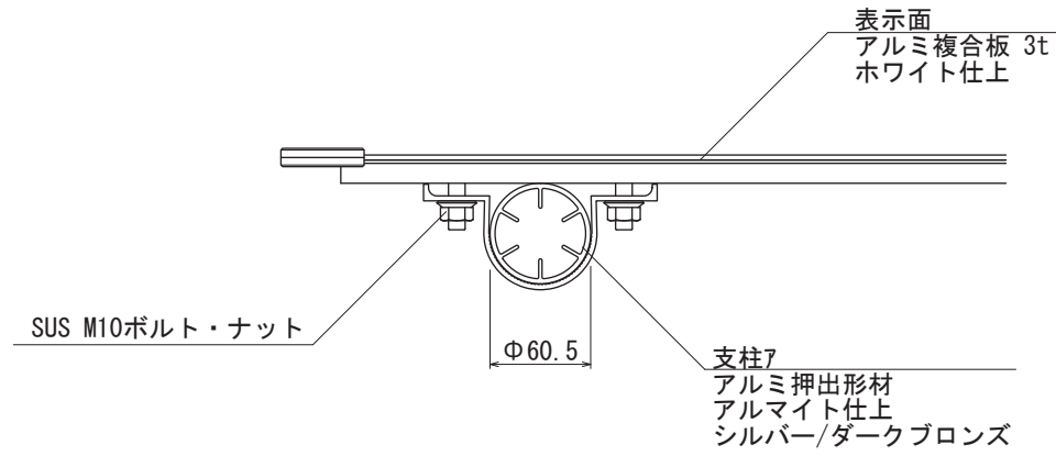
【平面図 S=1:5】
