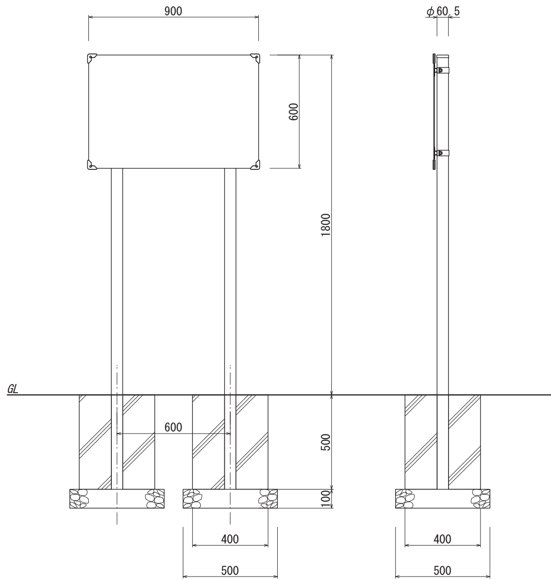
【正面図 S=1:20】
