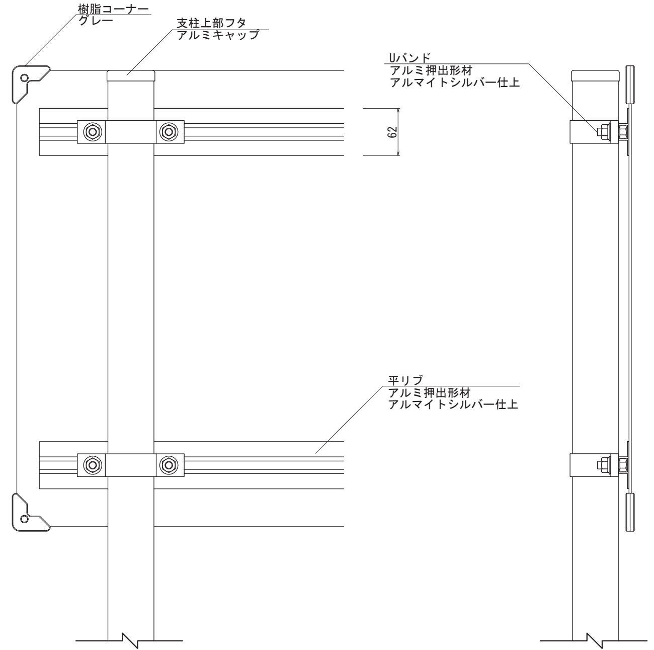
【背面図 S=1:5】
