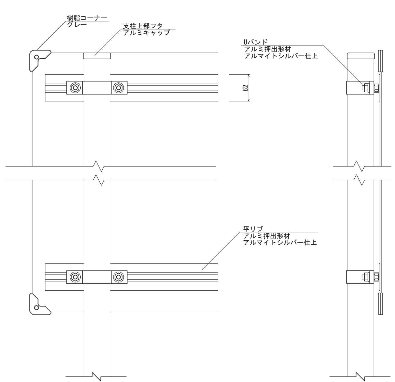
【背面図 S=1:5】
