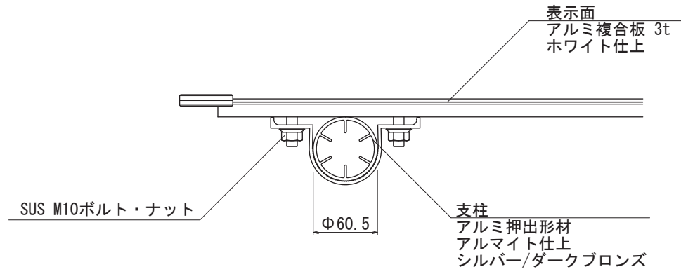
【平面図 S=1:5】
