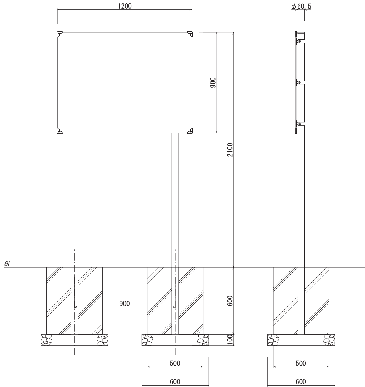
【正面図 S=1:20】
