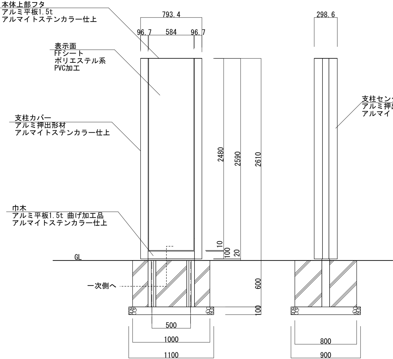
【正面図 S=1:30】
