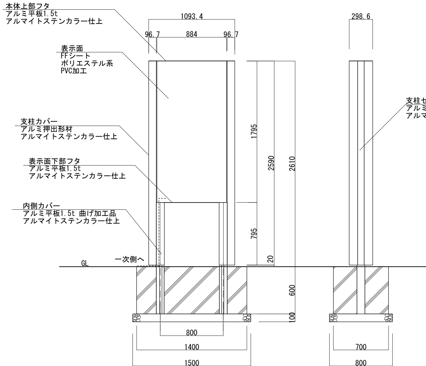
【正面図 S=1:30】
