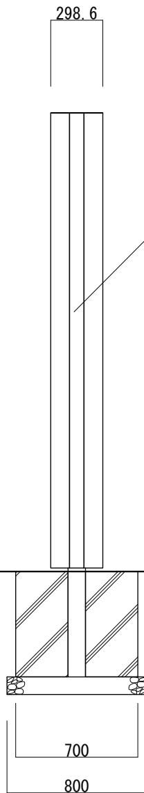
【側面図 S=1:30】
