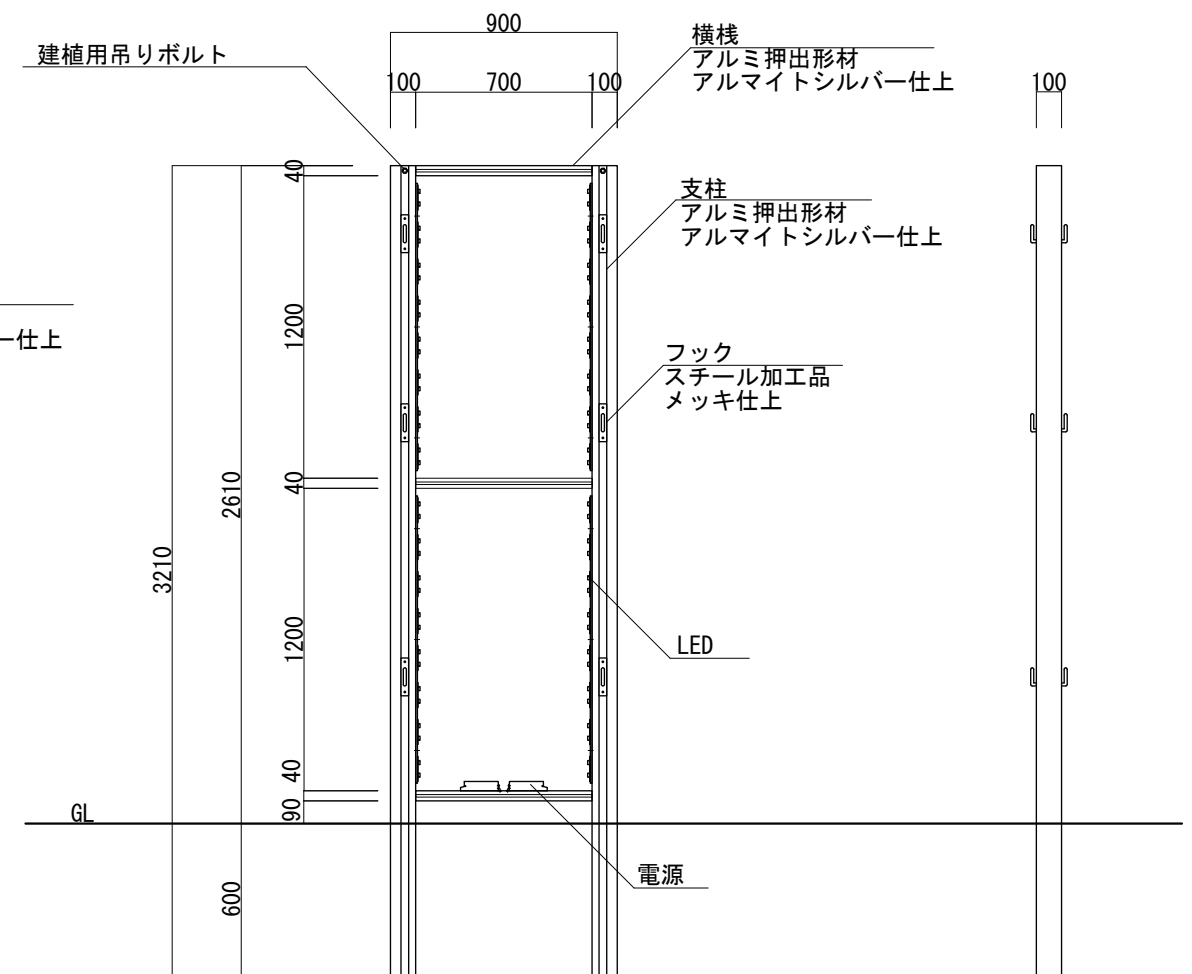
【フレーム正面図 S=1:30】
