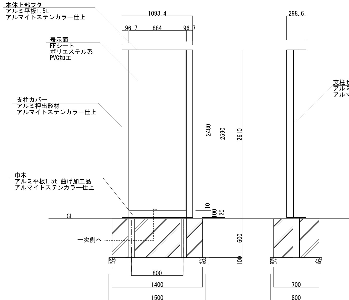
【正面図 S=1:30】
