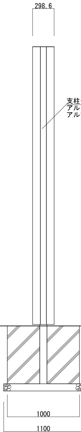
【側面図 S=1:30】
