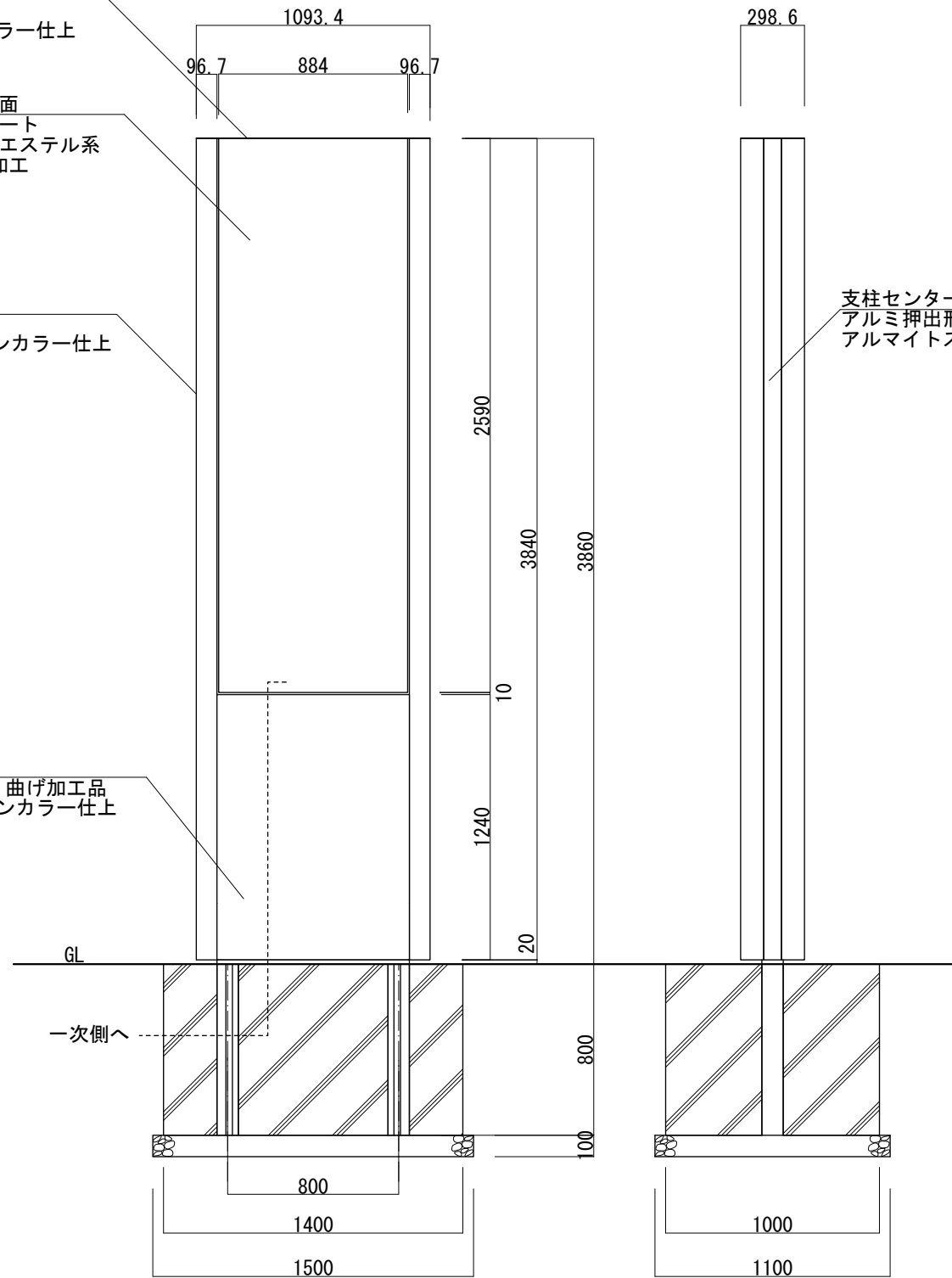
【正面図 S=1:30】
