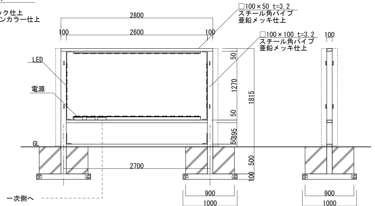
【鉄骨正面図 S=1:40】
