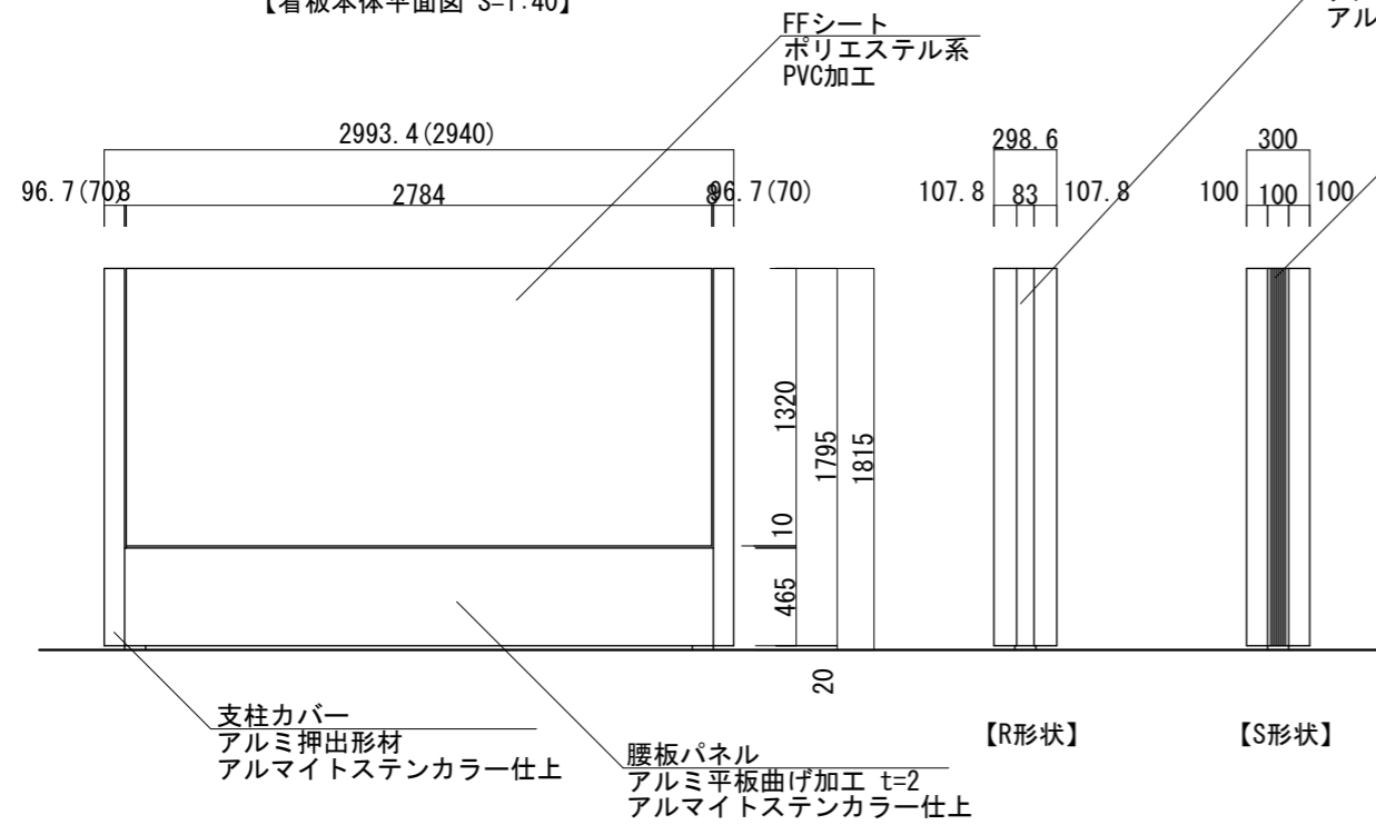
【看板本体正面図 S=1:40】
