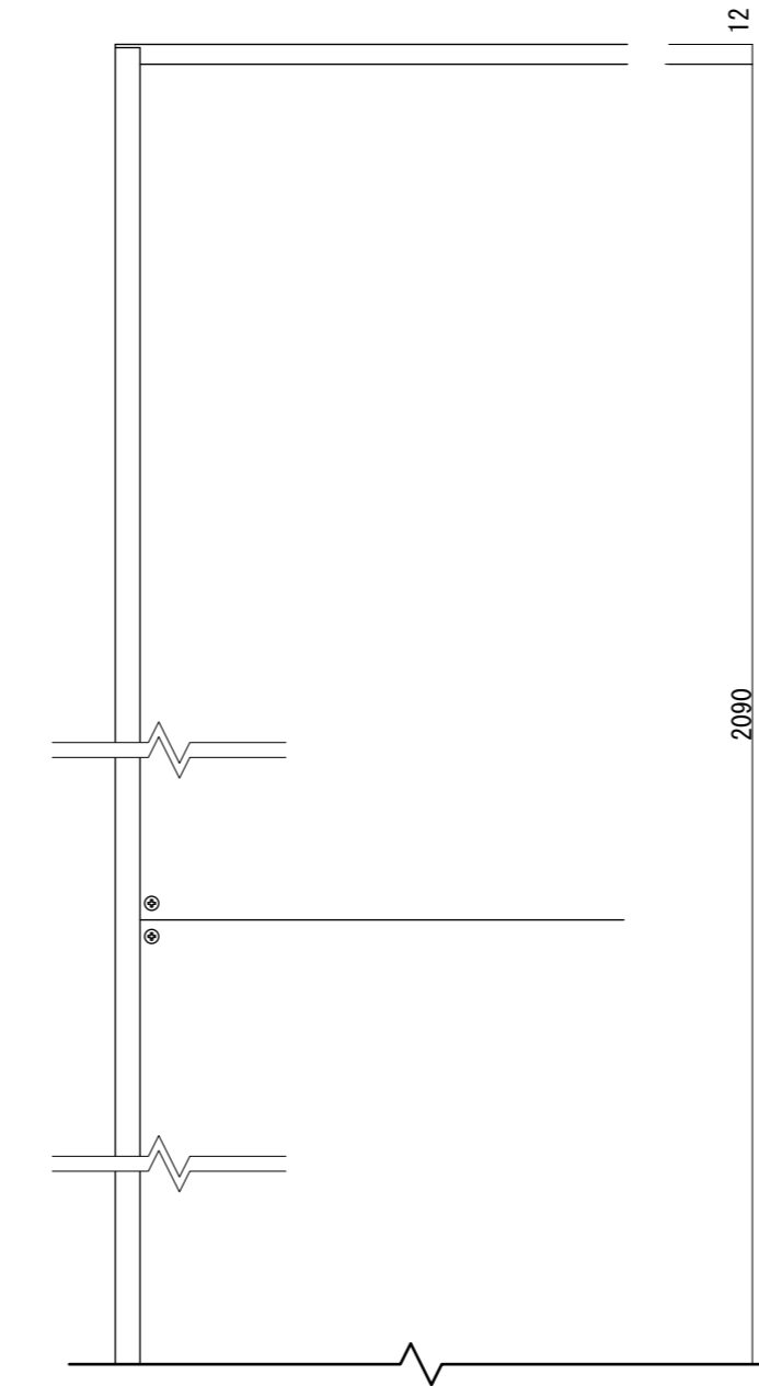
【正面図 S=1:5】
