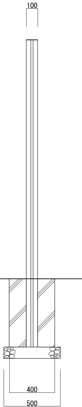
【側面図 S=1:20】
