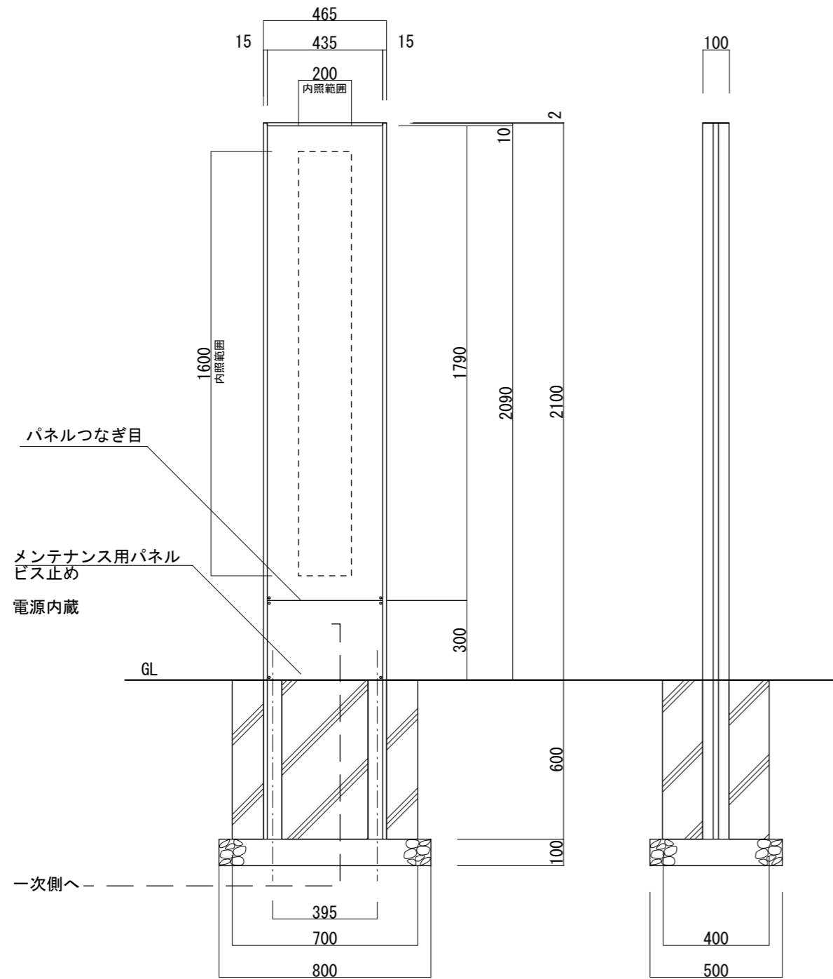
【正面図 S=1:20】
