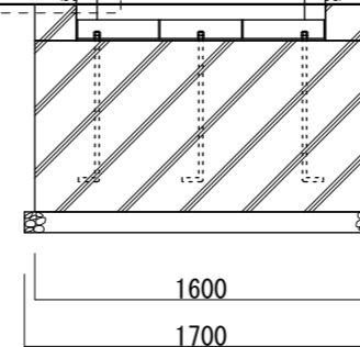
【鉄骨正面図 S=1:40】
