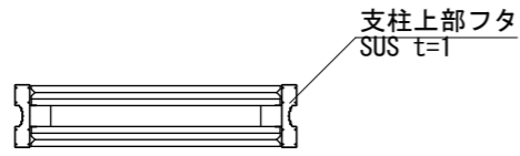
【平面図 S=1:40】
