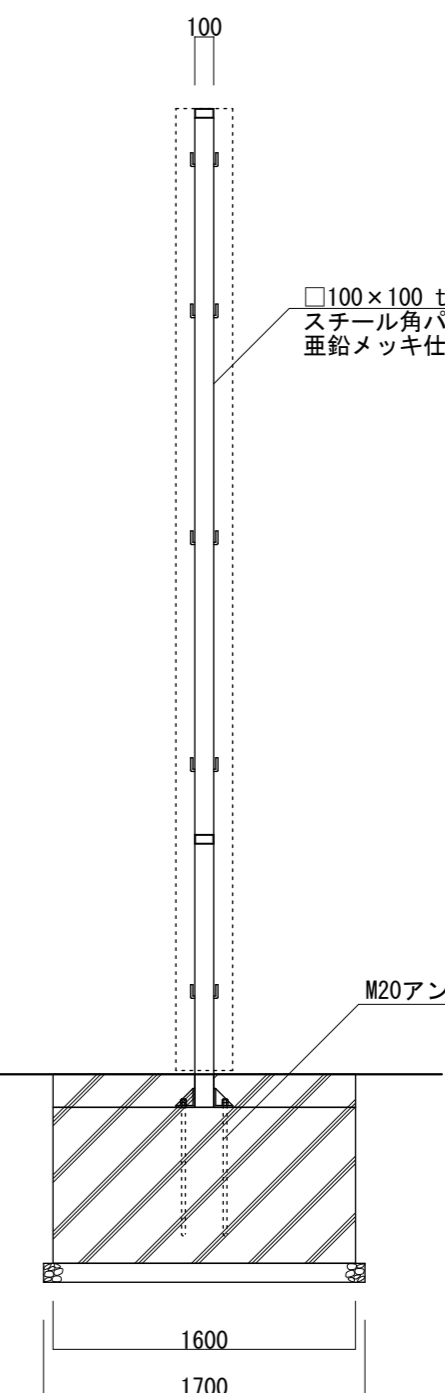
【鉄骨断面図 S=1:40】
