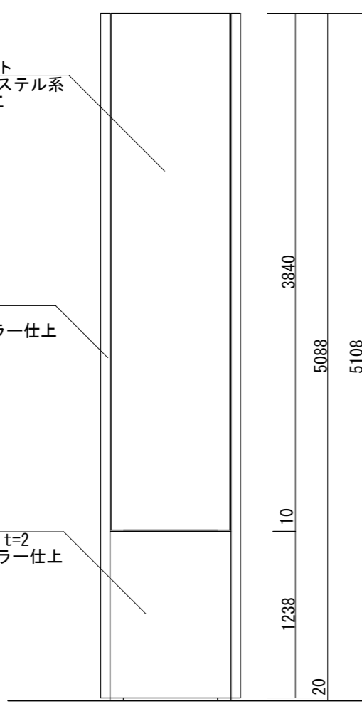
【正面図 S=1:40】
