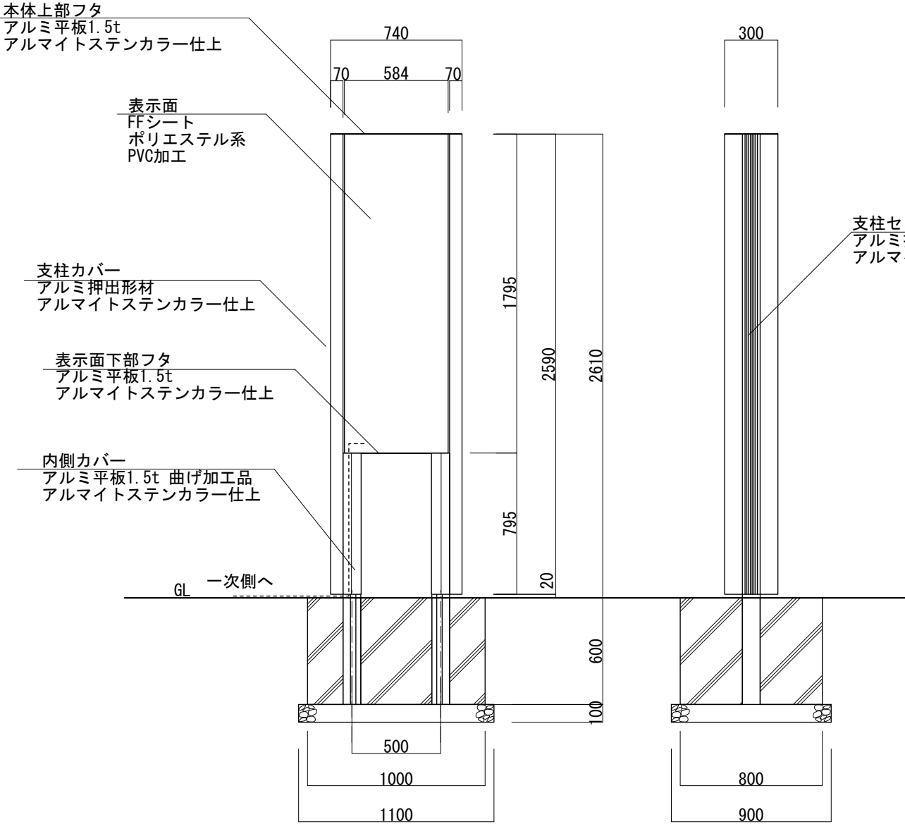
【正面図 S=1:30】
