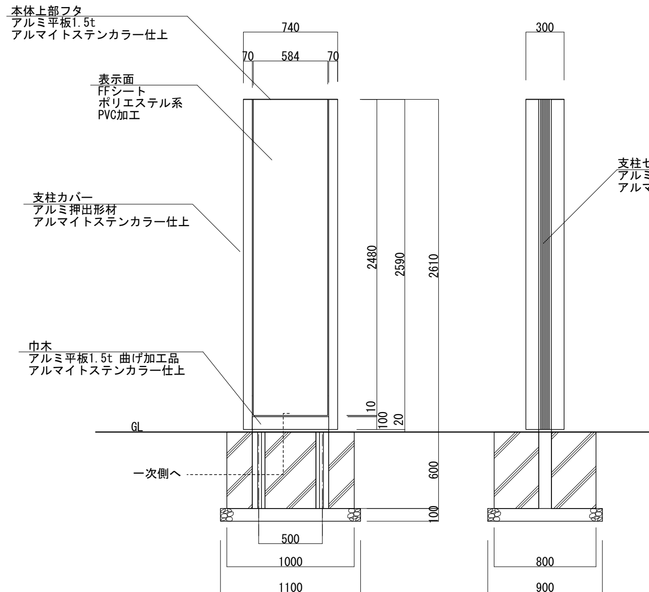
【正面図 S=1:30】
