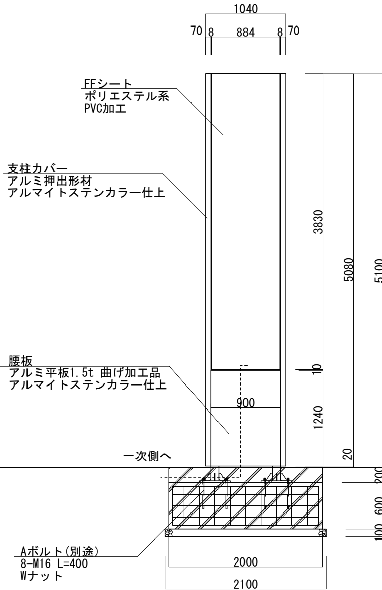
【正面図 S=1:50】
