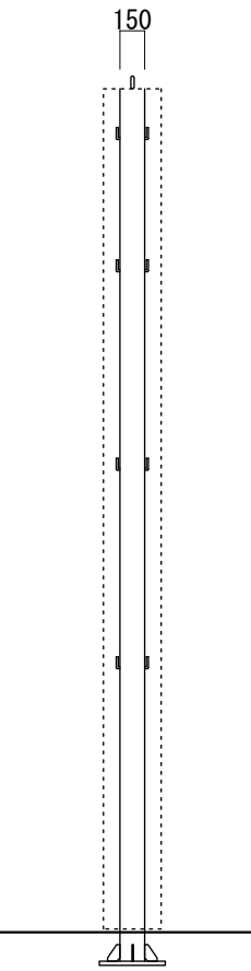
【鉄骨側面図 S=1:50】
