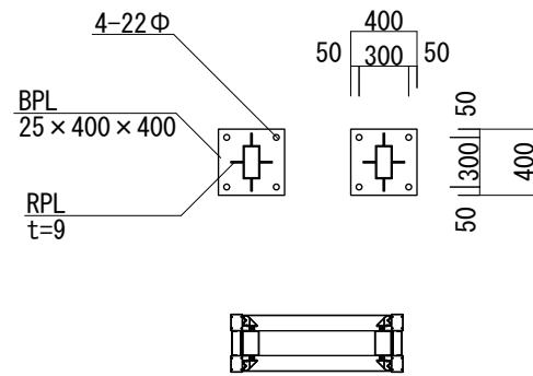
【断面図 S=1:50】
