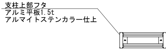
【平面図 S=1:50】
