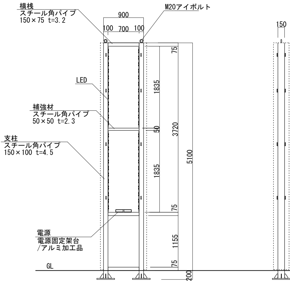
【鉄骨正面図 S=1:50】
