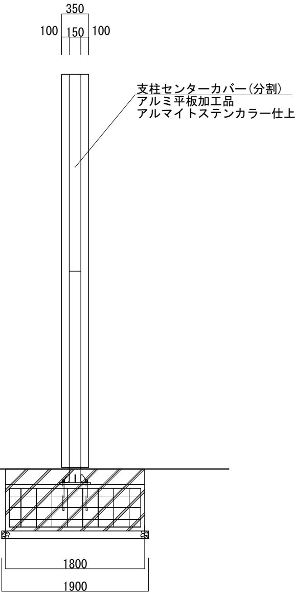
【側面図 S=1:50】
