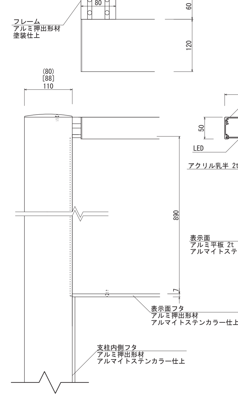
【正面図 S=1:5】
