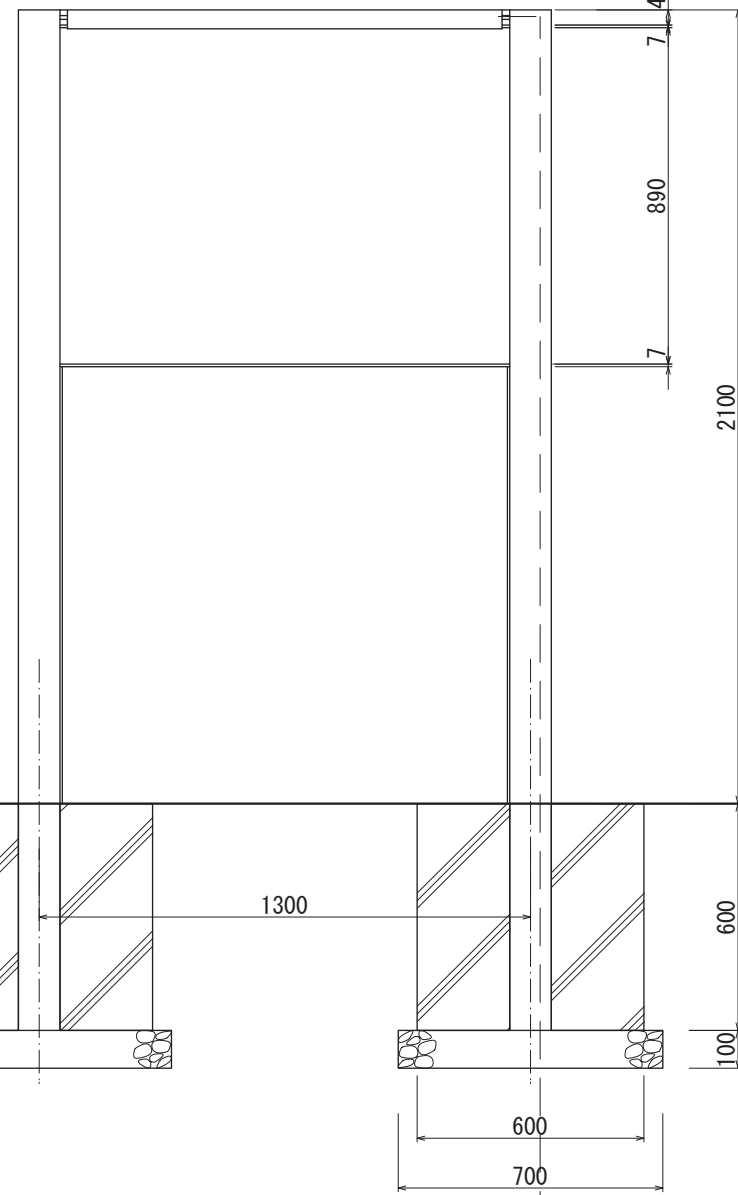
【正面図 S=1:20】
