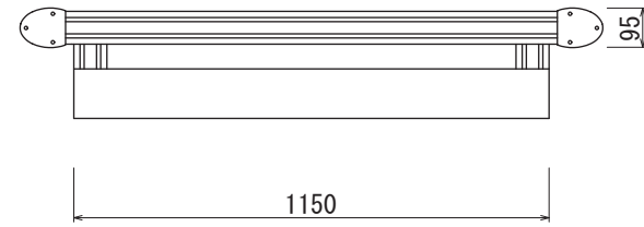
【平面図 S=1:20】
