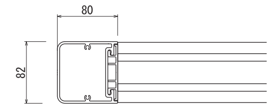
(S支柱)
