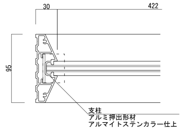
【平面図 S=1:3】
