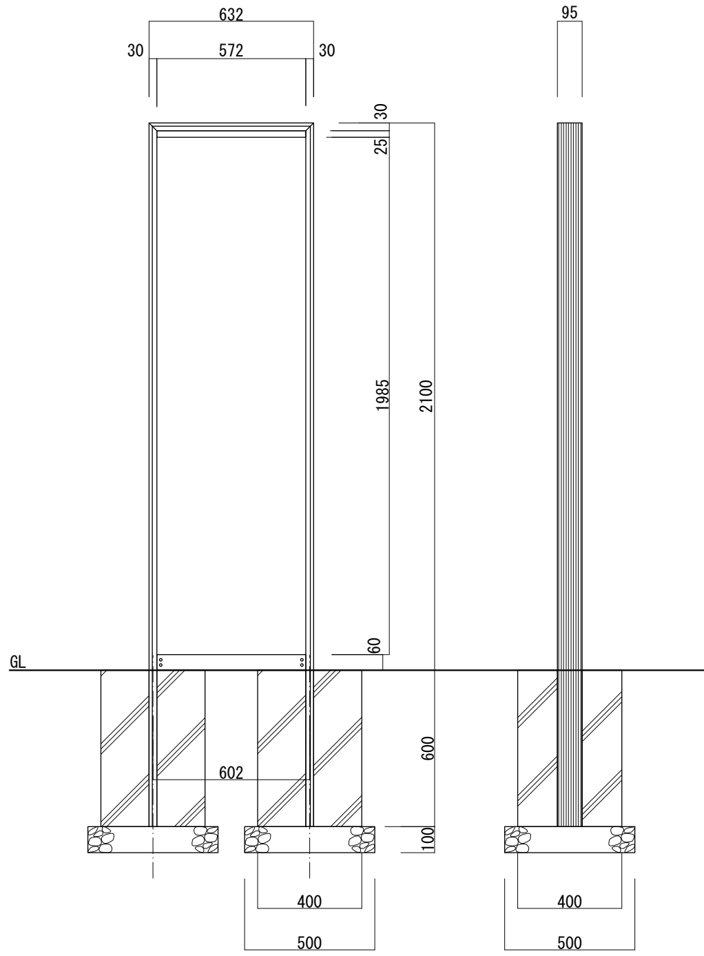
【正面図 S=1:20】
