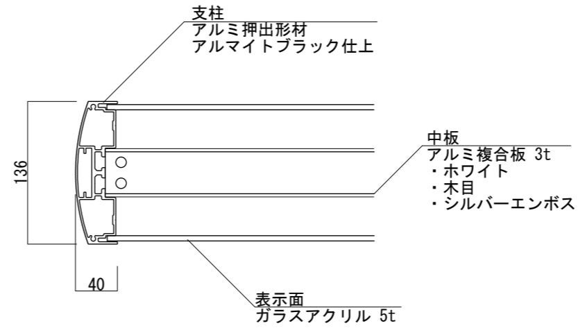
【平面図 S=1:5】
