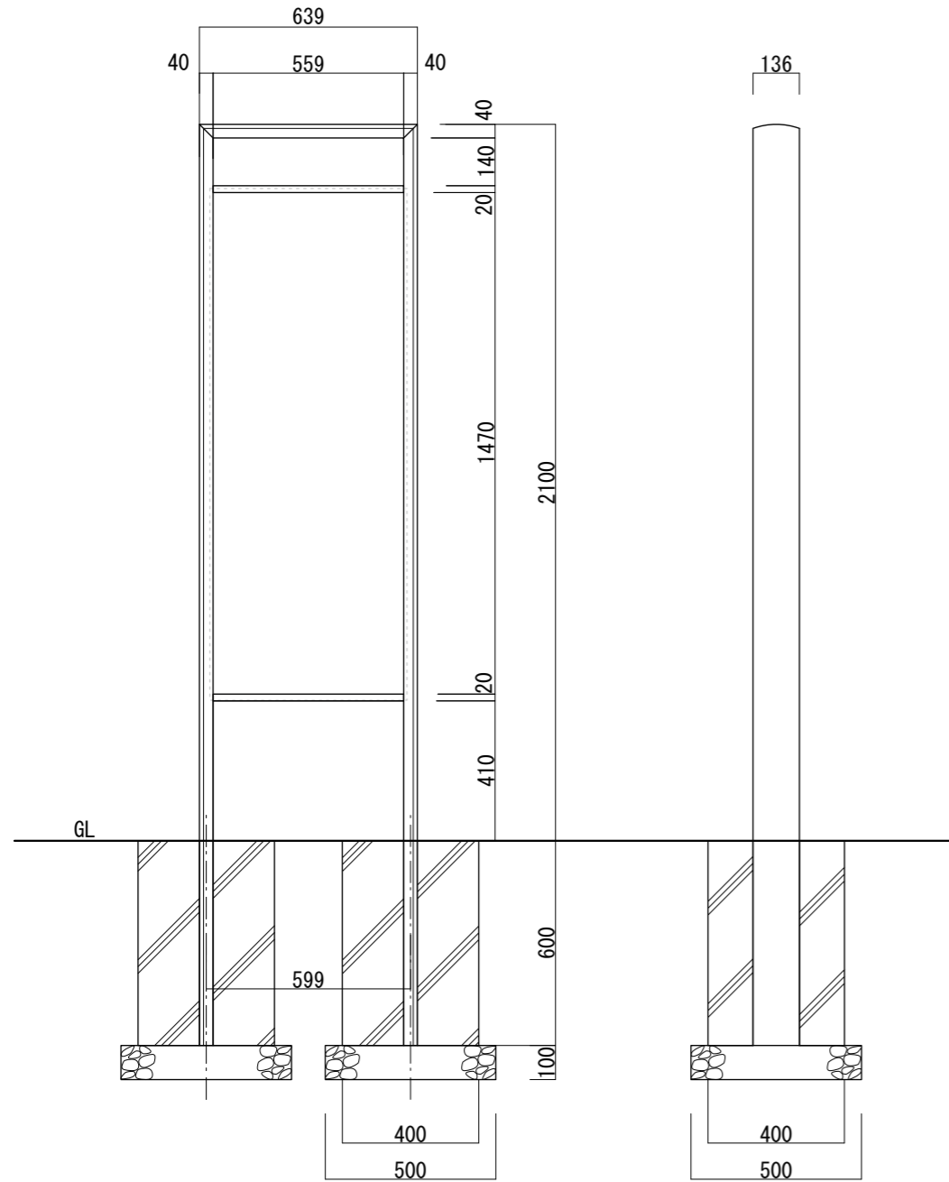
【正面図 S=1:20】
