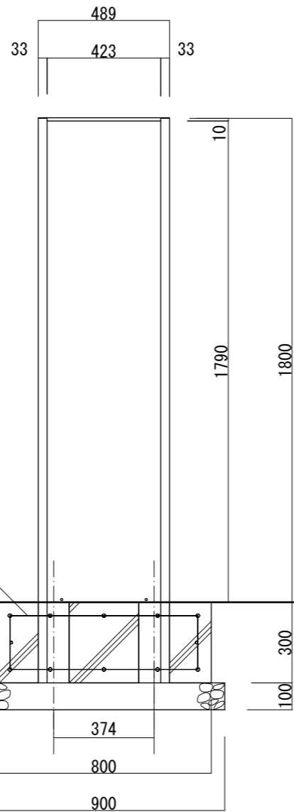
【側面図 S=1:20】
