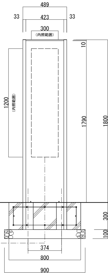
【正面図 S=1:20】
