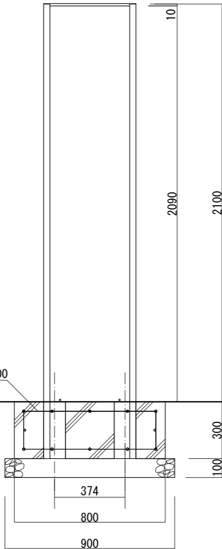
【側面図 S=1:20】
