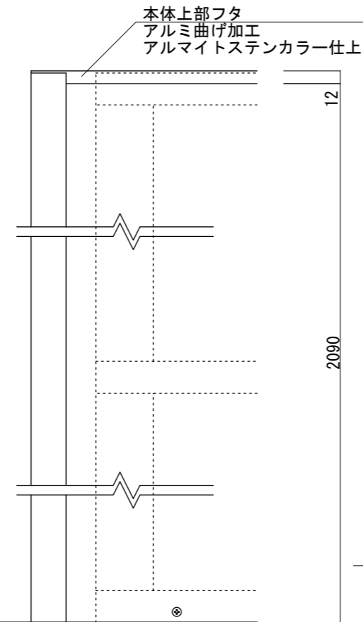
【正面図 S=1:5】
