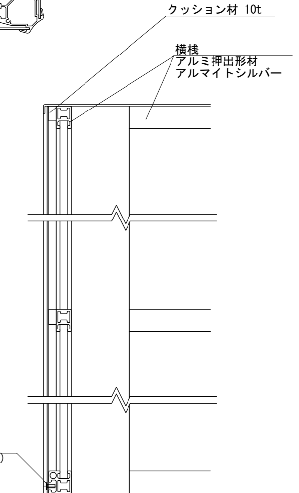
【断面図 S=1:5】
