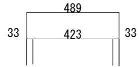
【平面図 S=1:20】
