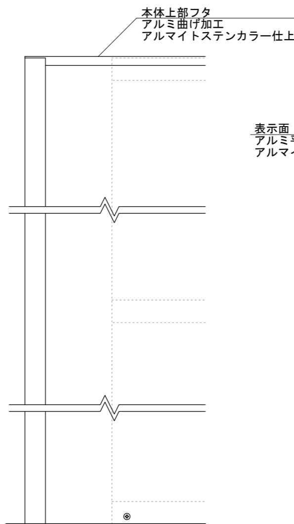
【正面図 S=1:5】
