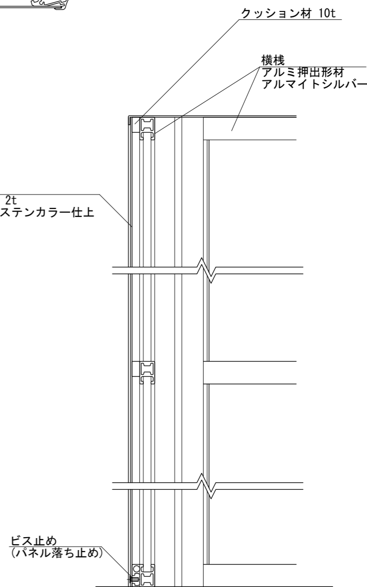
【断面図 S=1:5】
