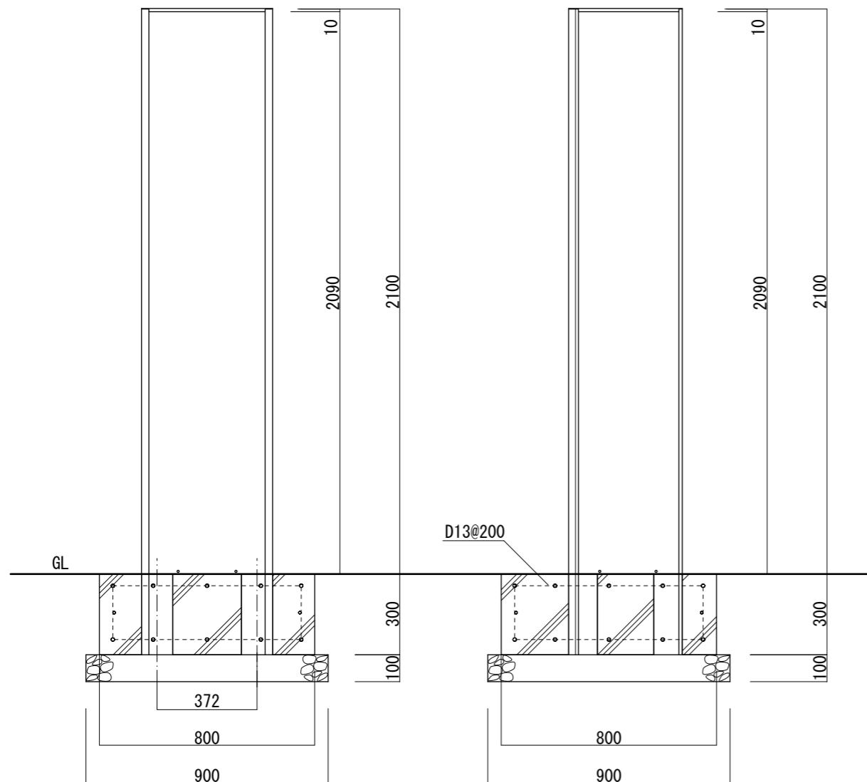
【正面図 S=1:20】
