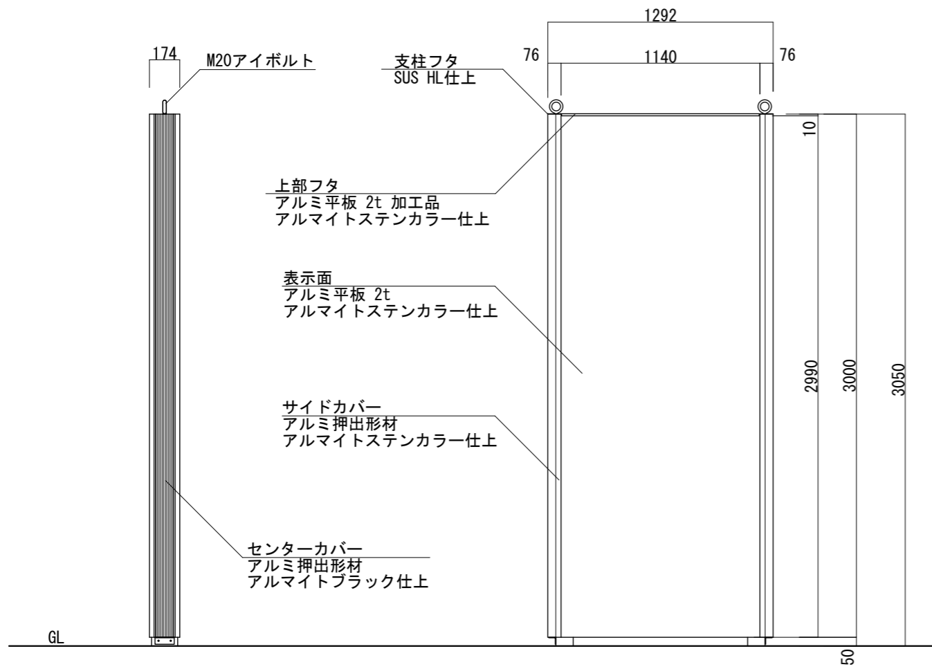
【側面図 S=1:30】
