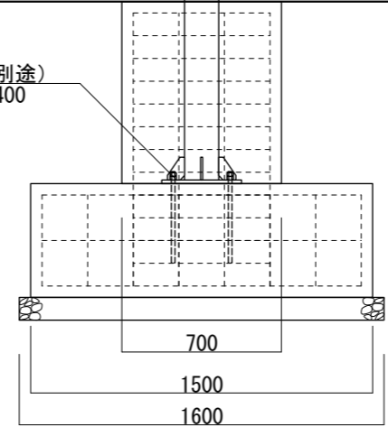
【鉄骨断面図 S=1:30】
