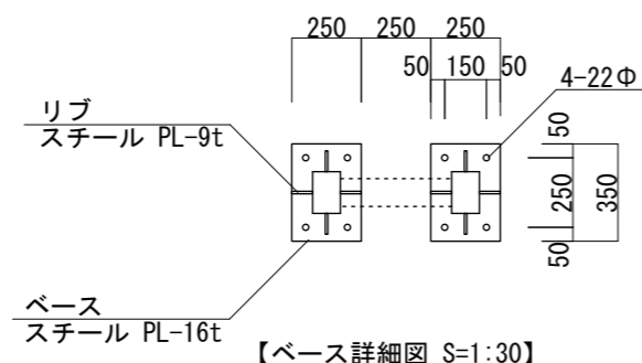
【ベース詳細図 S=1:30】
