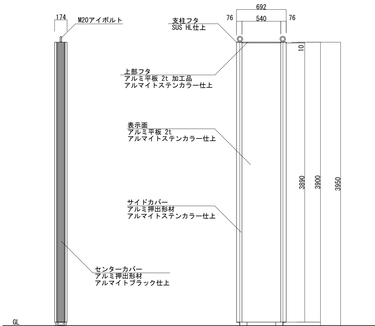
【側面図 S=1:30】
