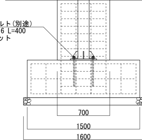
【鉄骨断面図 S=1:30】
