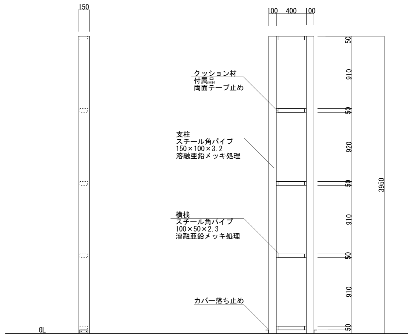
【断面図 S=1:30】
