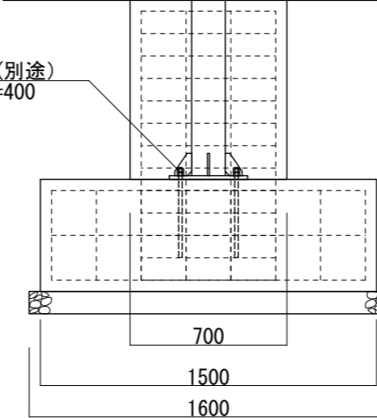
【鉄骨断面図 S=1:30】
