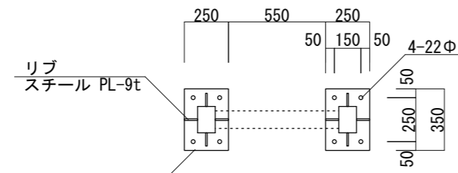
【ベース詳細図 S=1:30】
