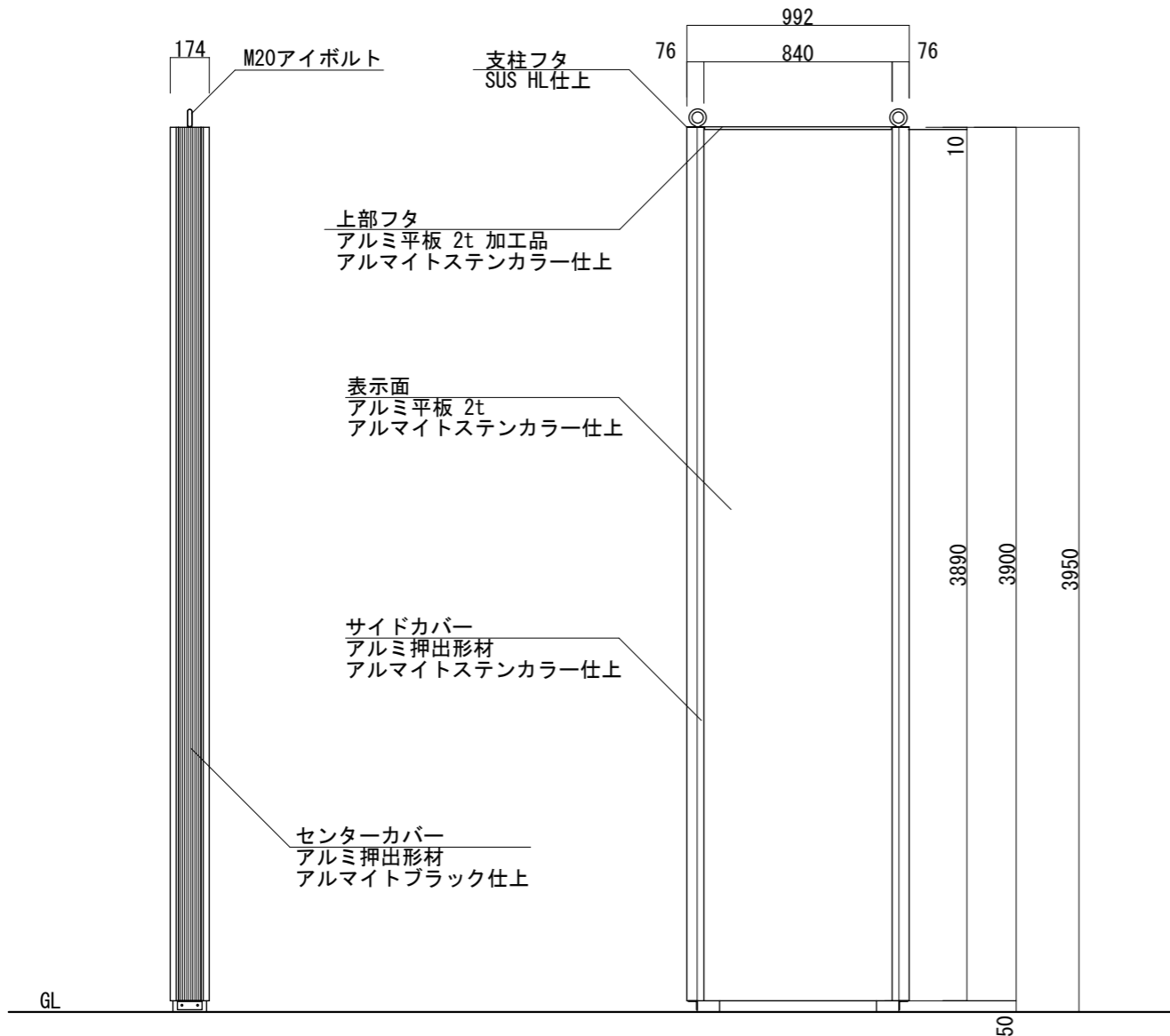
【側面図 S=1:30】
