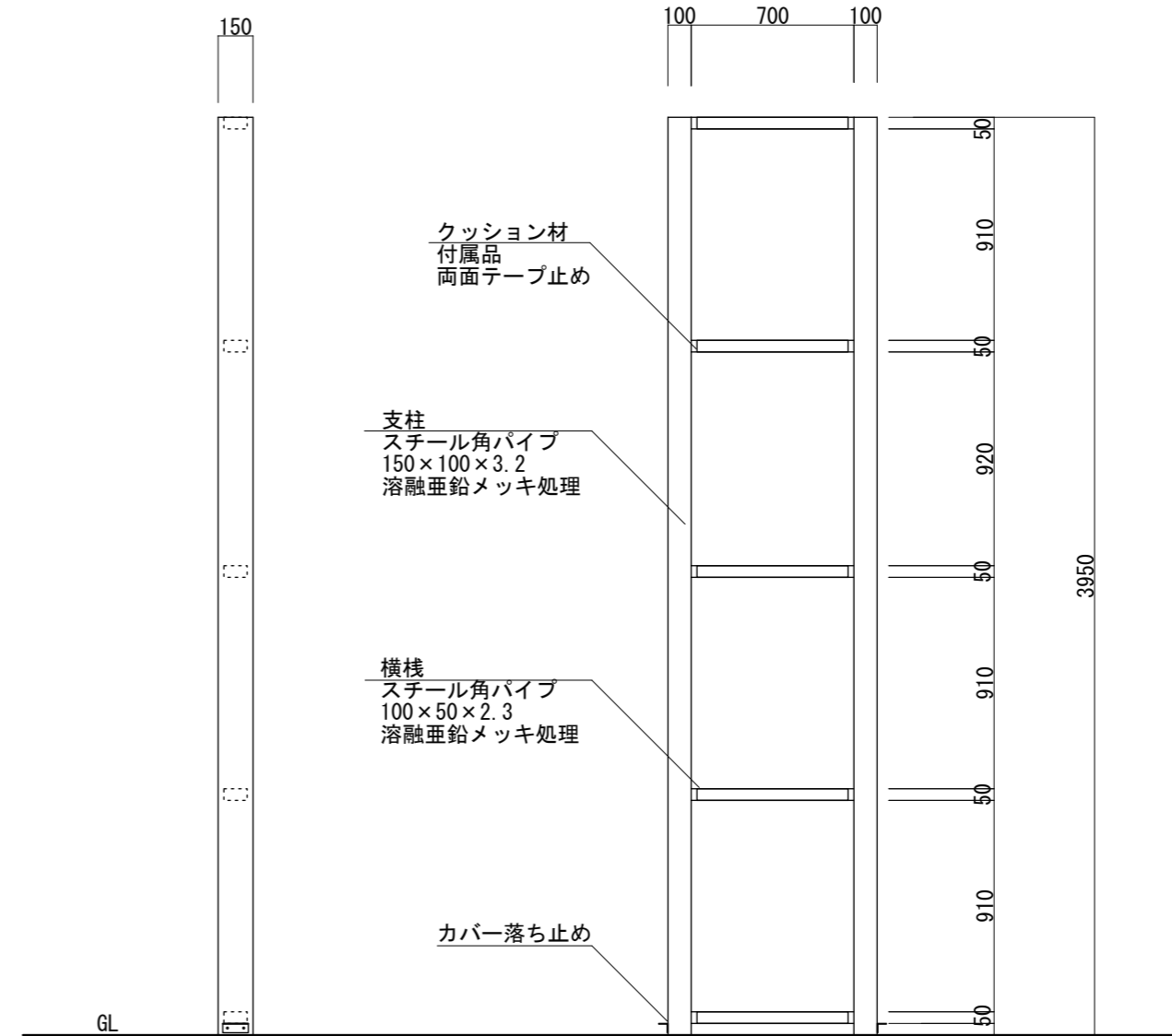
【断面図 S=1:30】
