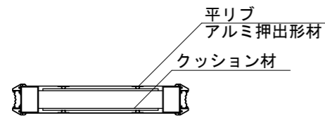
【断面図 S=1:30】
