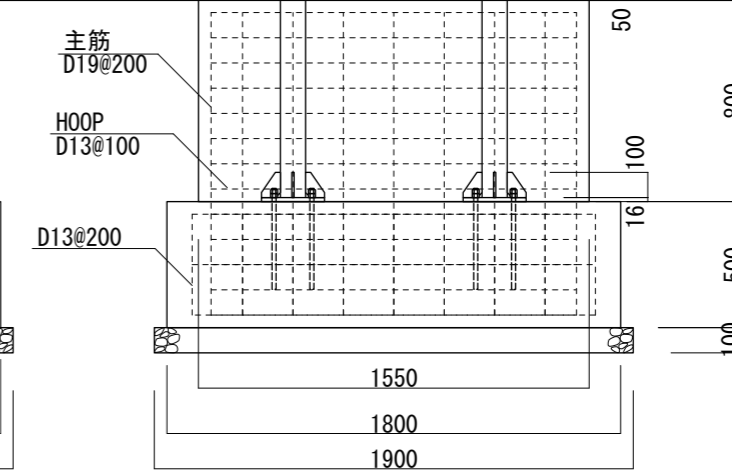
【鉄骨正面図 S=1:30】
