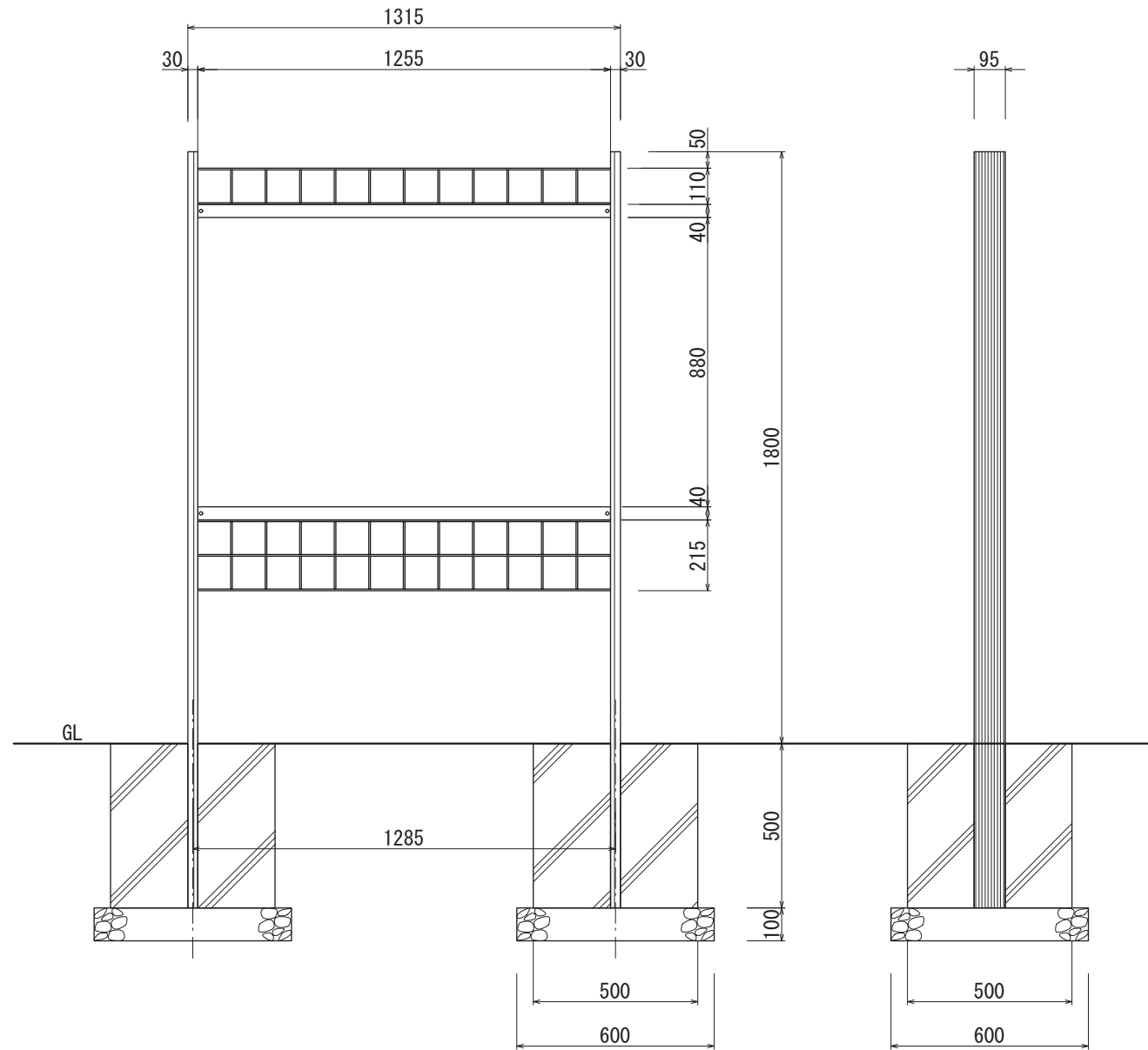
【正面図 S=1:20】
