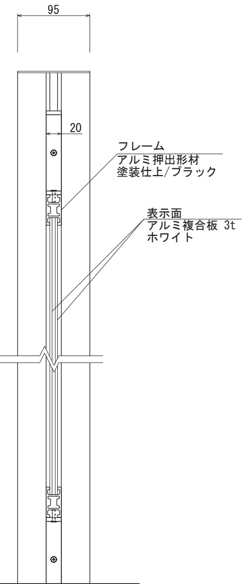
【側面図 S=1:5】
