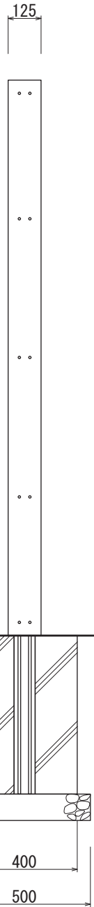
【側面図 S=1:20】
