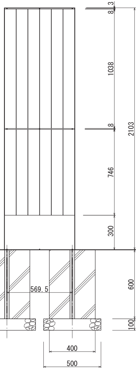
【正面図 S=1:20】
