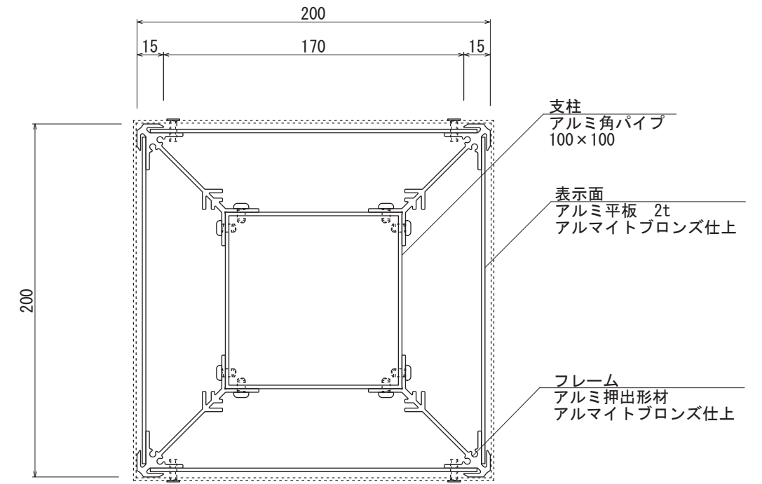
【断面図 S=1:3】
