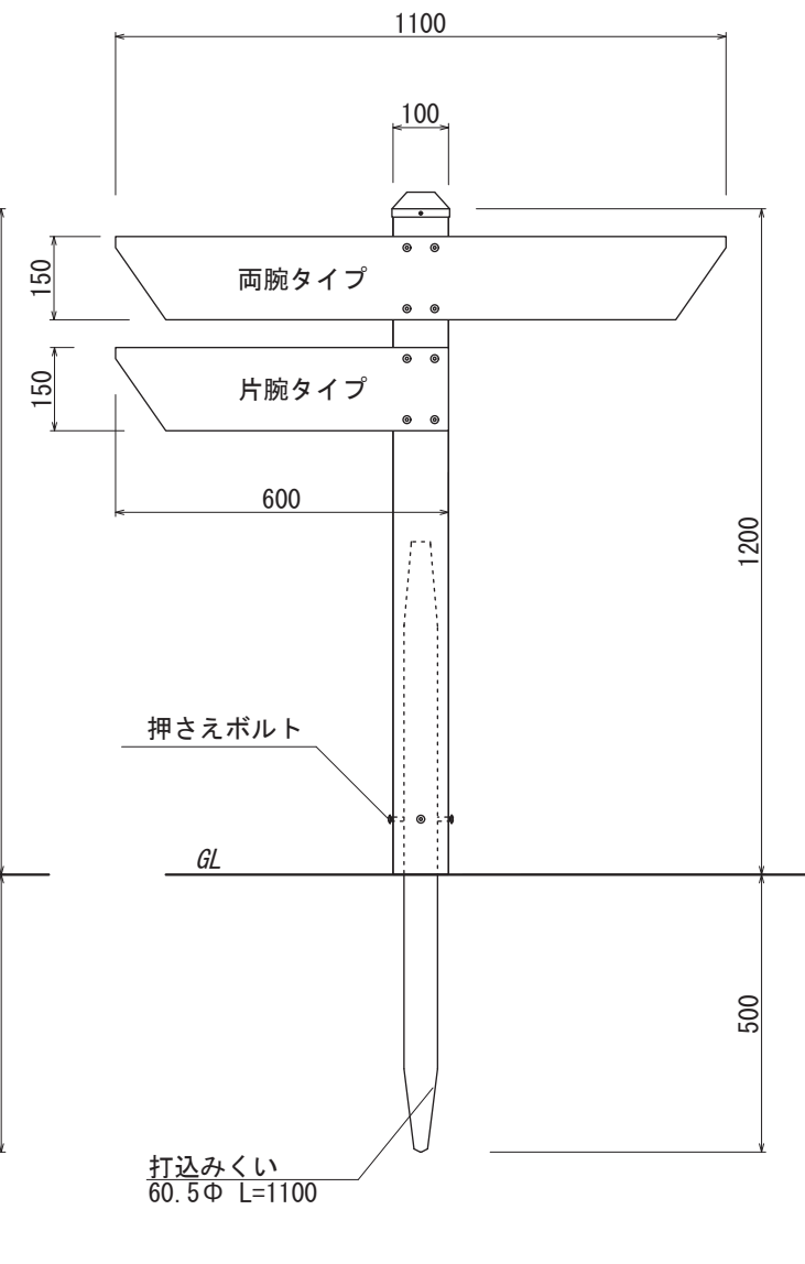
【打込みくいタイプ】
