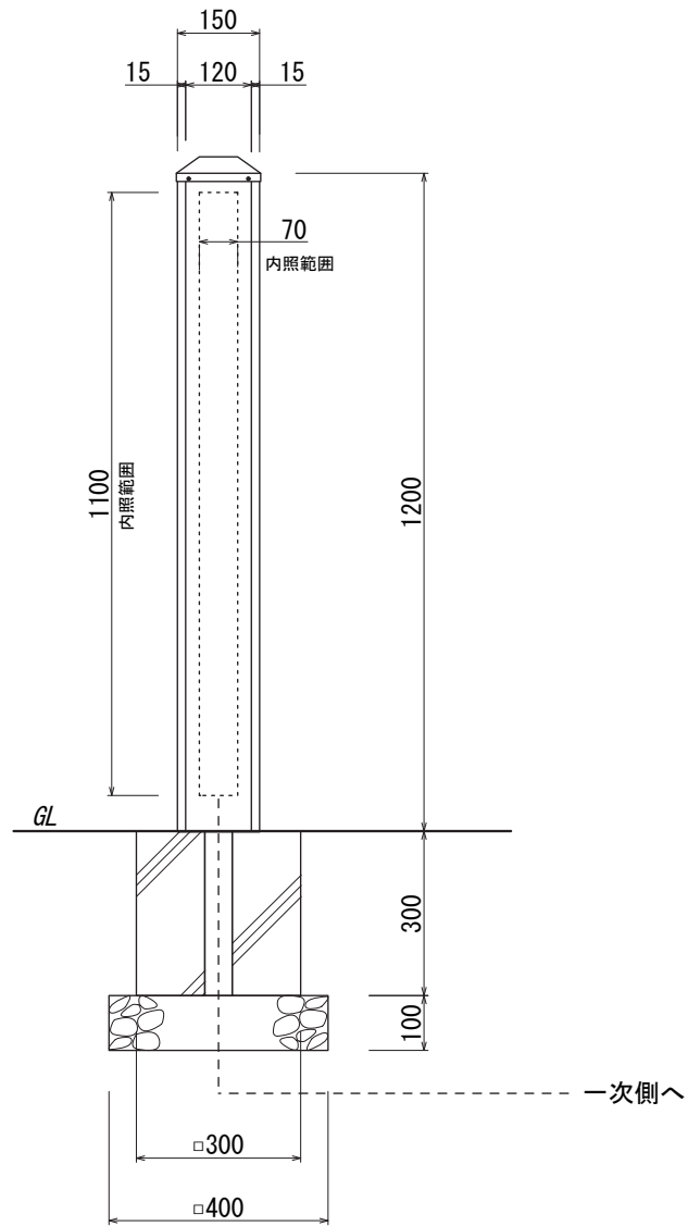
【正面図 S=1:15】
