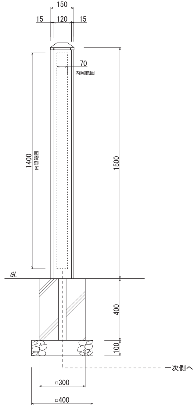
【正面図 S=1:15】
