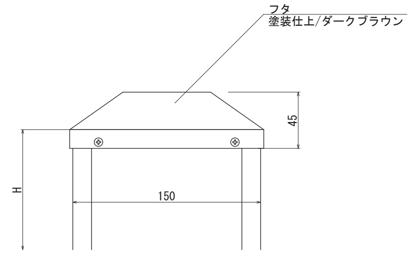
【正面図 S=1:3】
