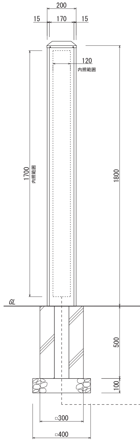
【正面図 S=1:15】
