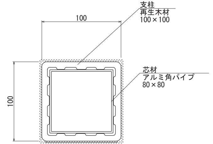
【断面図 S=1:3】
