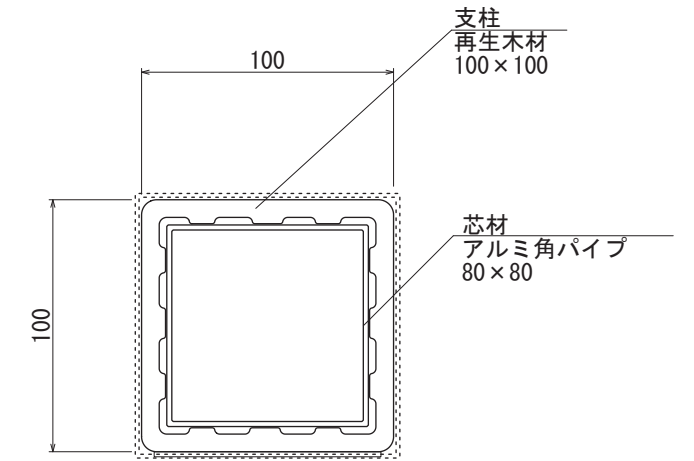
【断面図 S=1:3】
