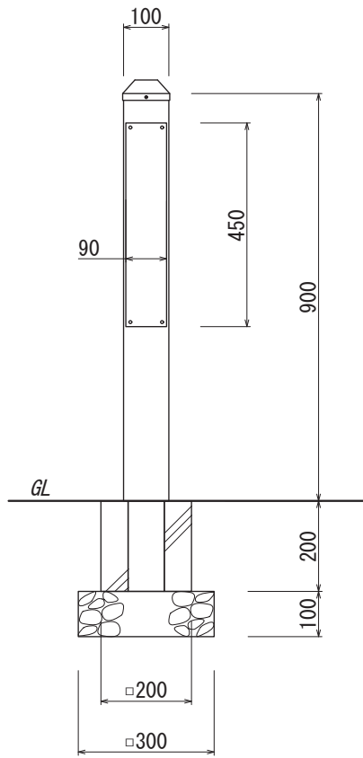
【基礎タイプ】
