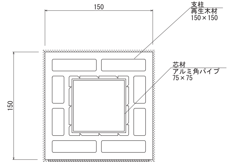
【断面図 S=1:3】
