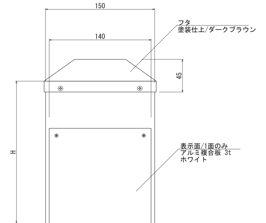
【正面図 S=1:3】
