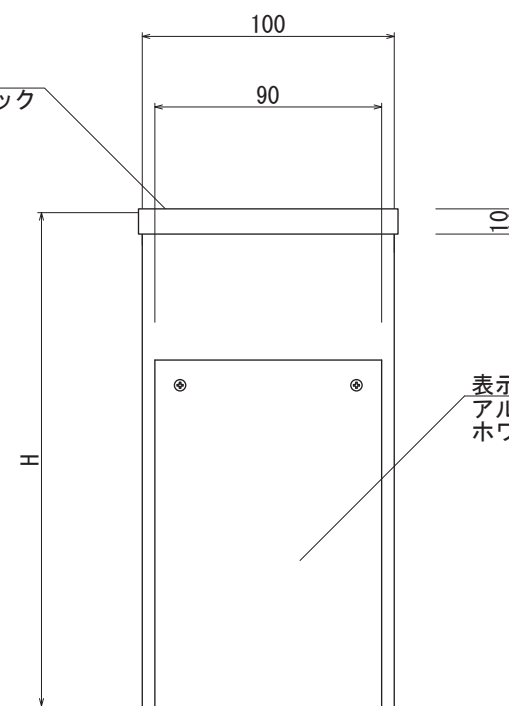
【正面図 S=1:3】
