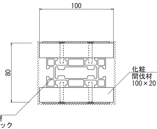
【断面図 S=1:3】
