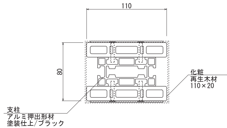
【断面図 S=1:3】
