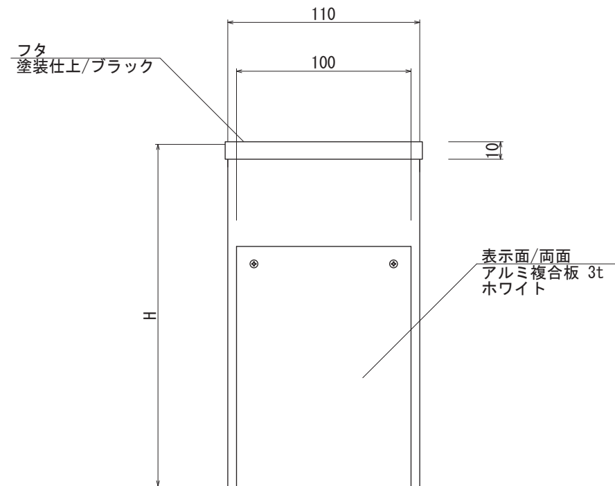
【正面図 S=1:3】
